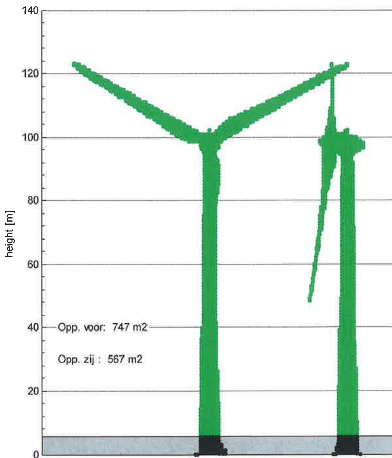
Figuur 5. Enercon E101 met ashoogte 99 m. Van zowel het voor- als zijaanzicht is de schaduwwerking berekend. Er is rekening gehouden met afscherming van de voet van het gebouw door het tussenliggende terrein.
