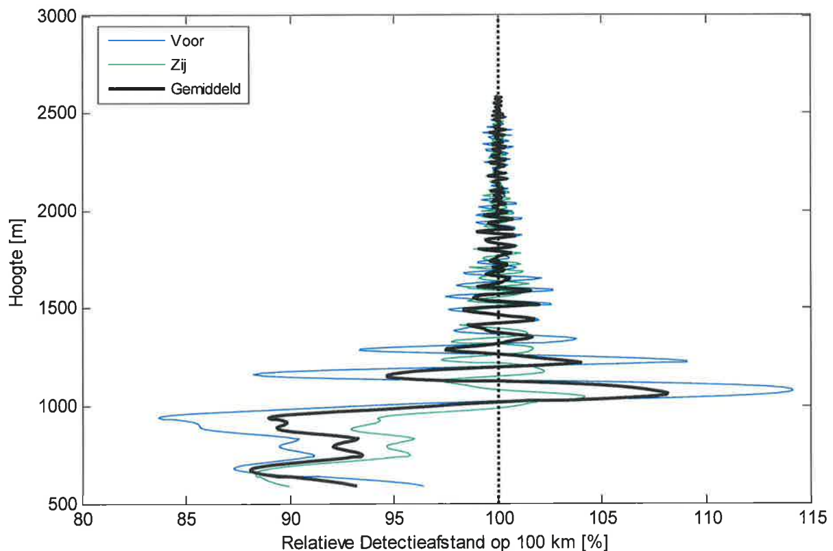
Figuur 6. Profielen van de relatieve detectieafstand als gevolg van het schaduw effect voor de windturbine van het type Enercon E101 met ashoogte 99 m.
