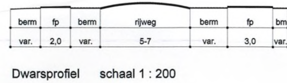
Dwarsprofiel schaal 1 : 200
