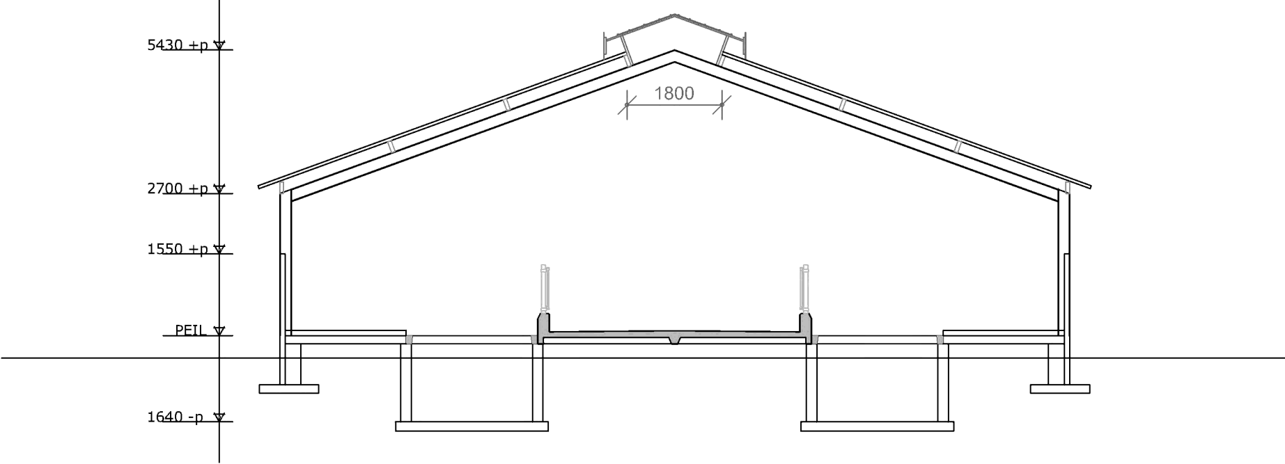
DOORSNEDE B-B
