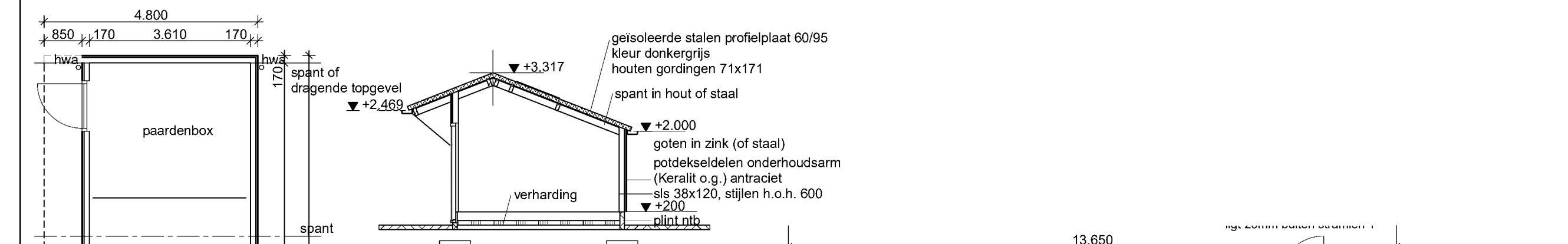
Doorsnede F-F
