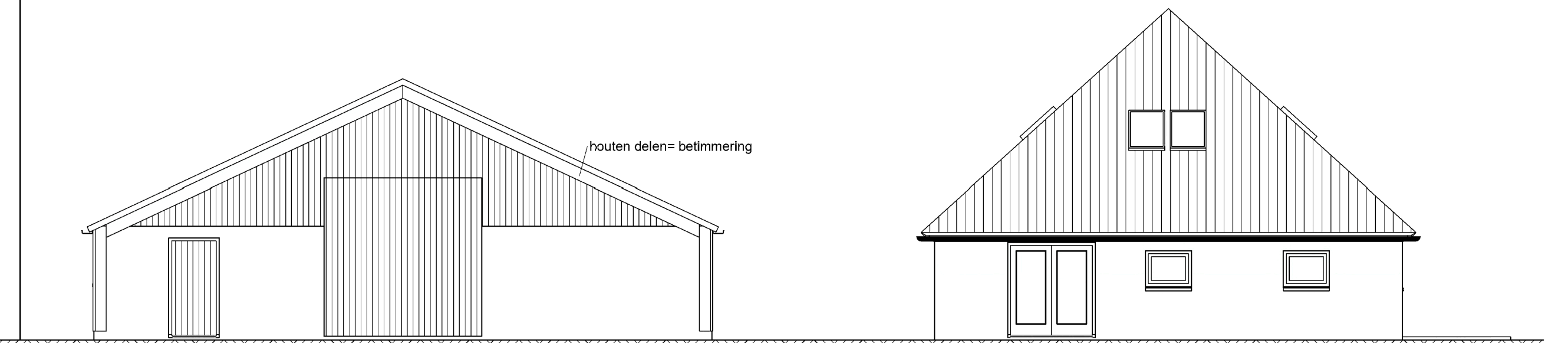
Achtergevel= noord
