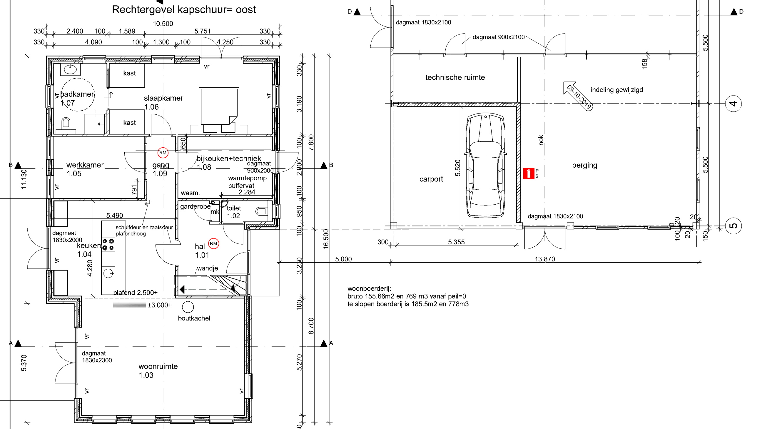
Begane grond
