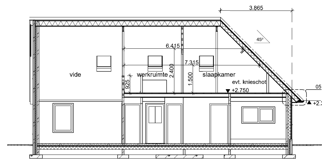
Doorsnede C-C
