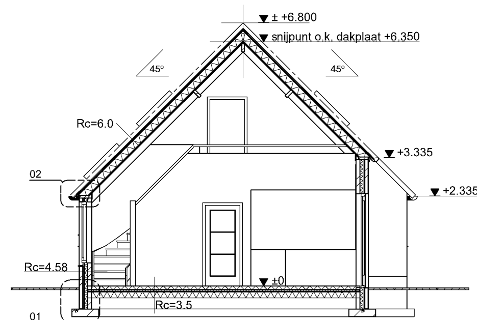
Doorsnede A-A
