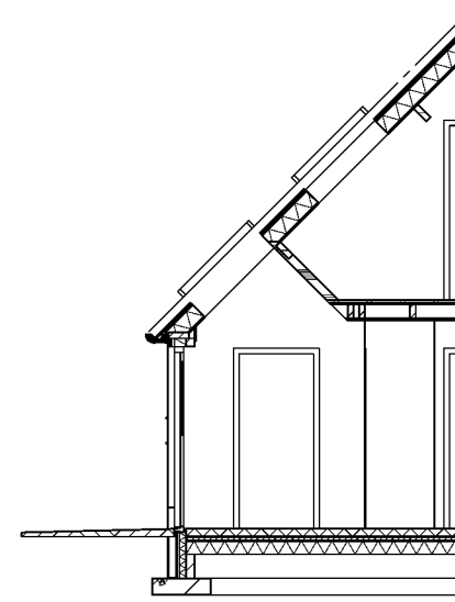
Doorsnede B1-B1
