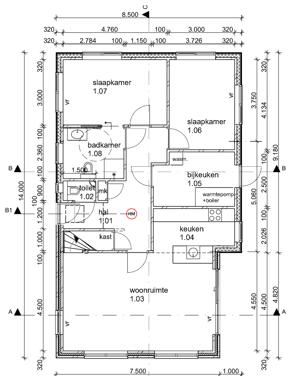
Begane grond
