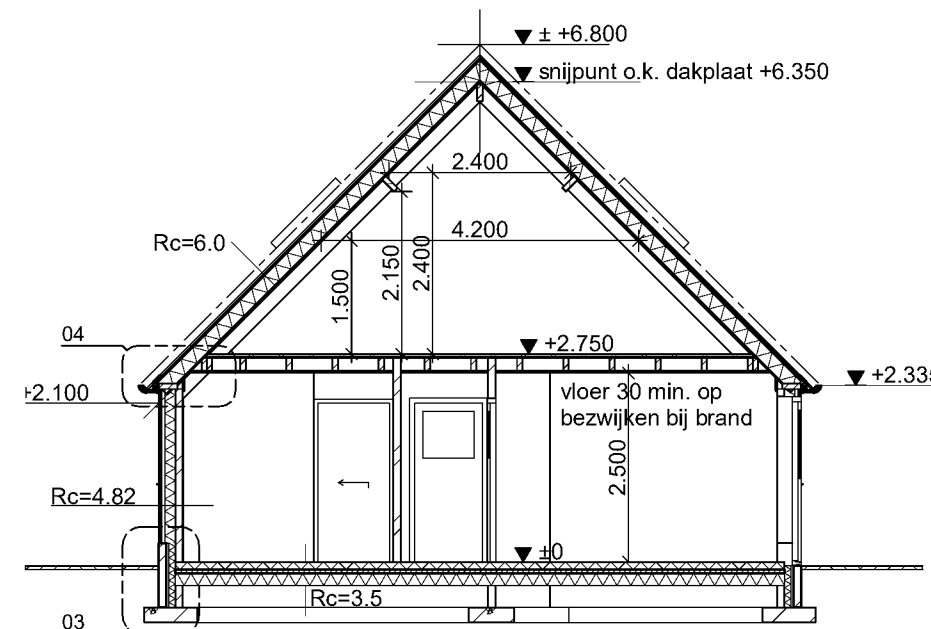
Doorsnede B-B
