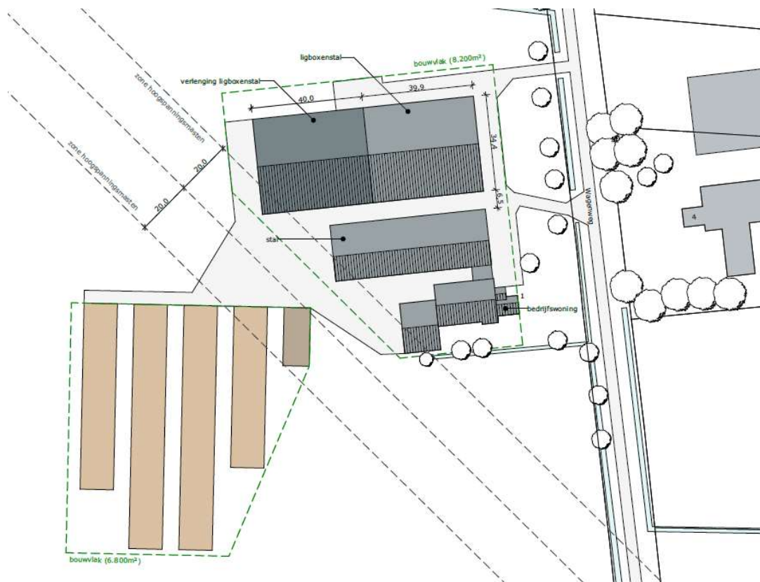
• Figuur 5: Situatietekening gewenste situatie Wagenweg 1 te Kuinre
