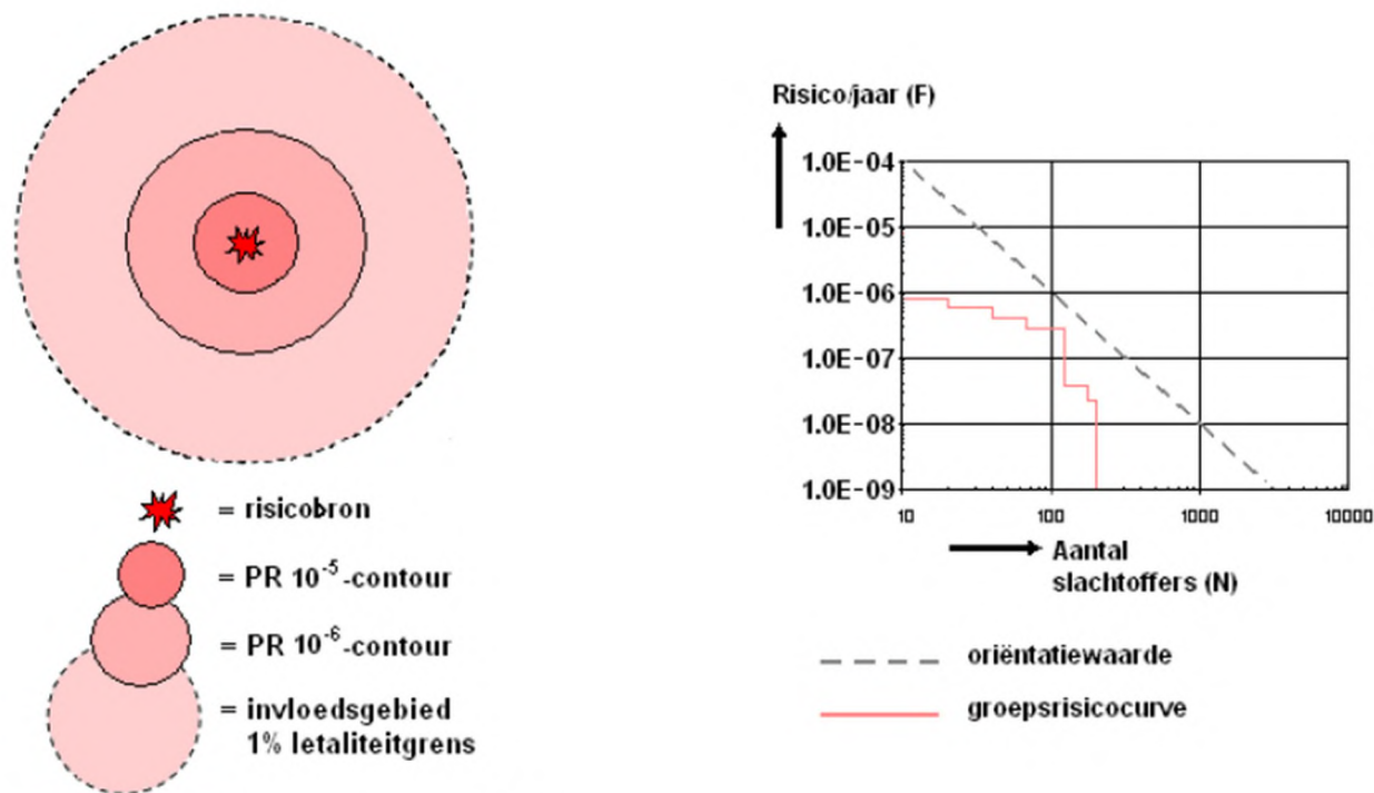
Afbeelding 4: Plaatsgebonden risicocontouren en fN-curve
