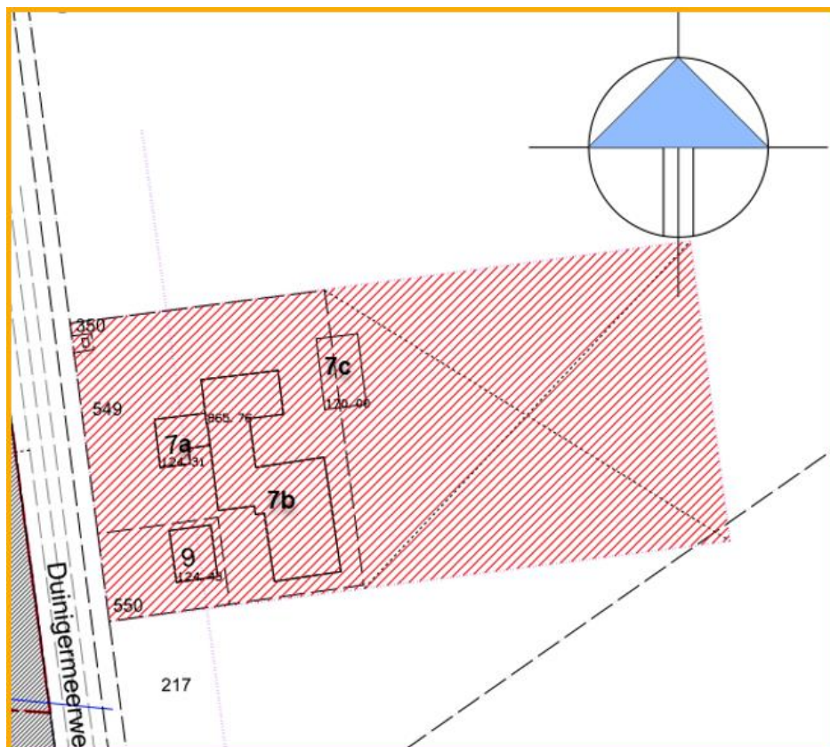
Figuur 1. Plantekening met de gewenste situatie van de nieuwe stal (E). De bestaande bebouwing bij de huisnummers 7 en 9 wordt verwijderd. Hiervoor komen drie woningen terug. (Bron: Bouwkundig Tekemburo Nico Bollen).
