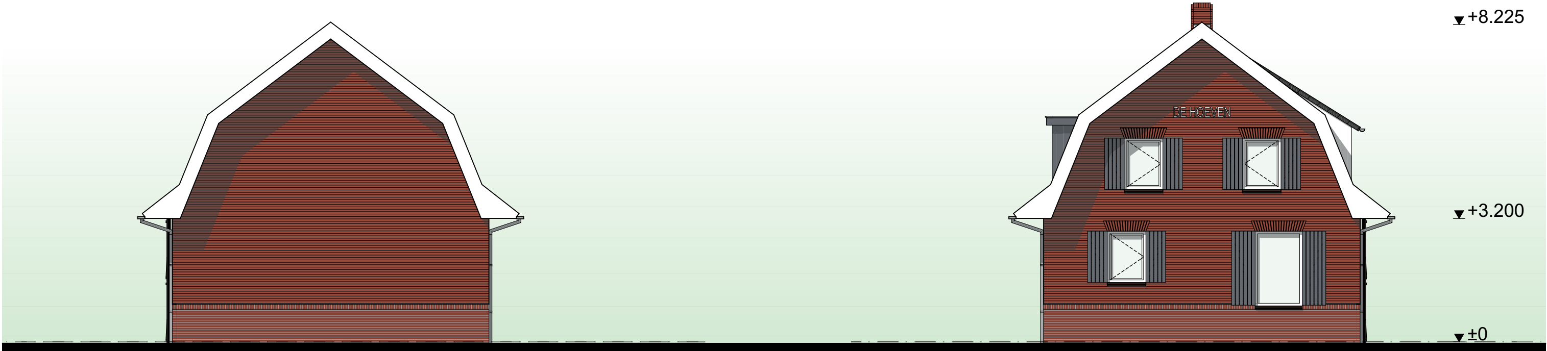
Rechtergevel (bestaand)
