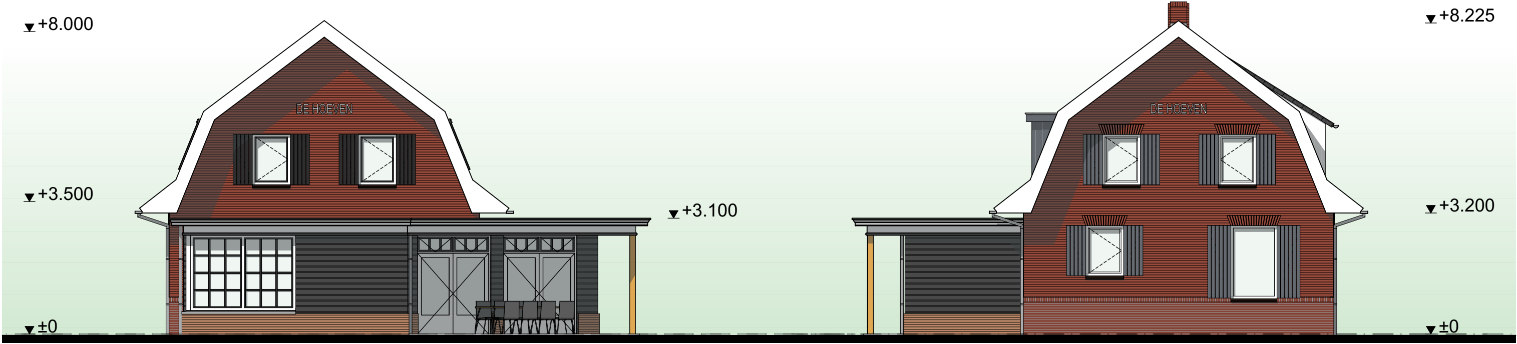
Rechtergevel (nieuw)
