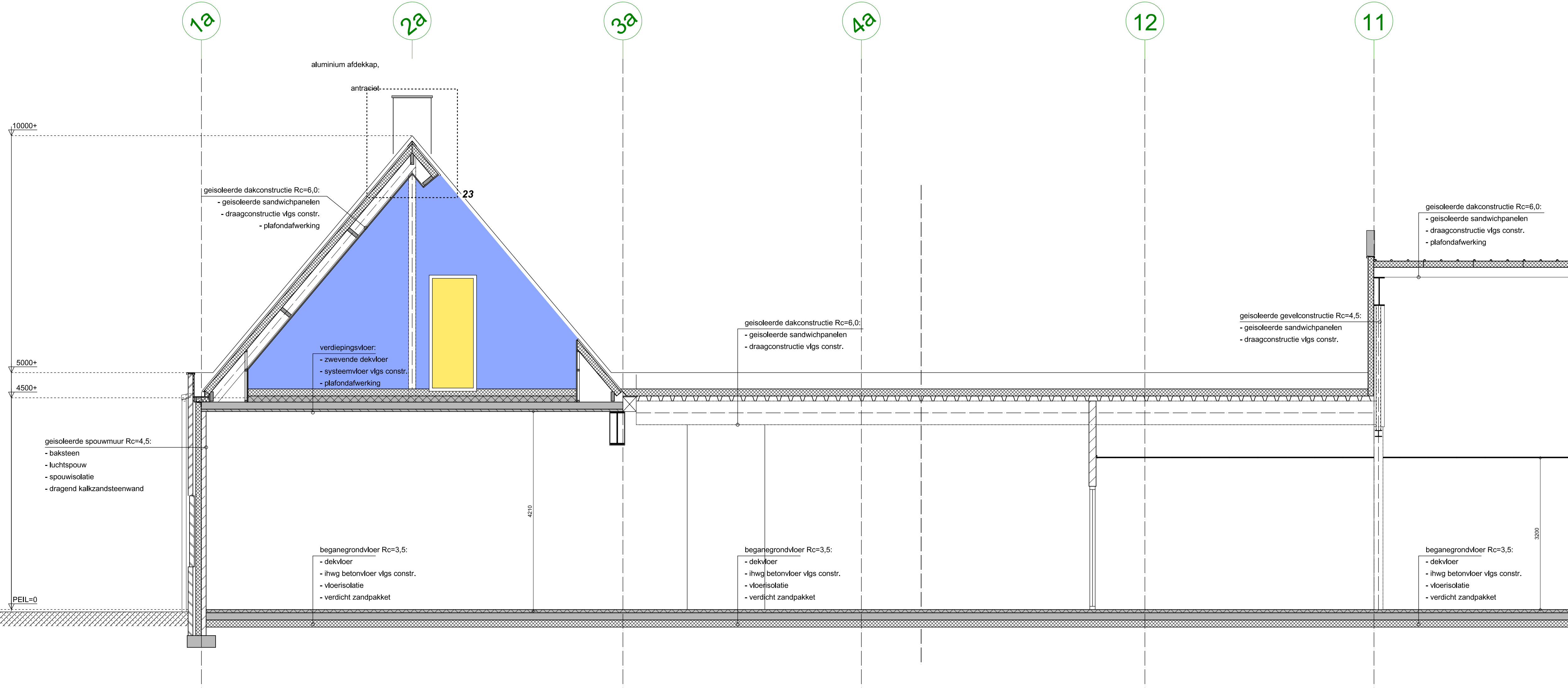
DOORSNEDE B-B
