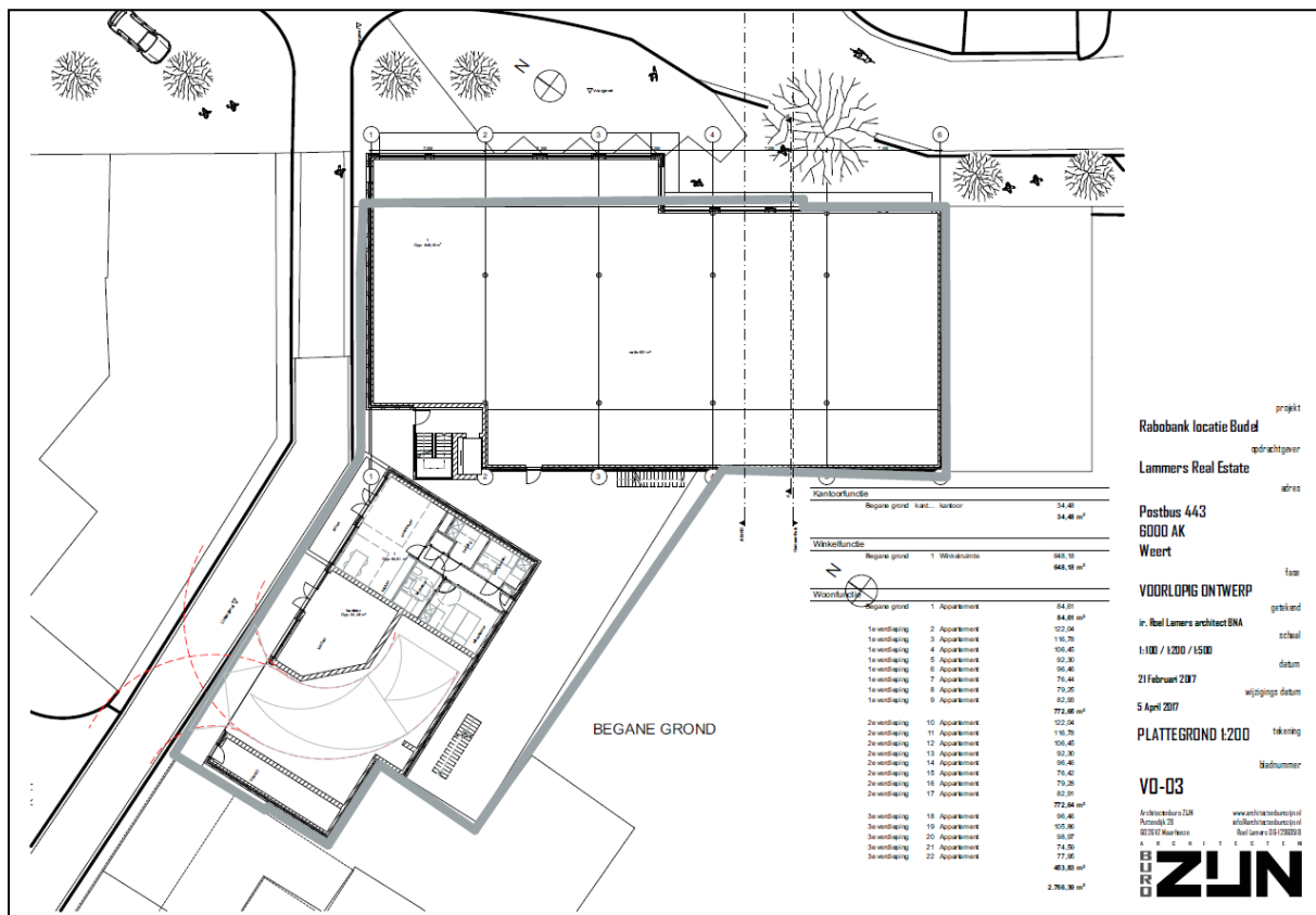
Figuur 9. Voorlopig ontwerp multifunctioneel gebouw Rabobank locatie Budel.
