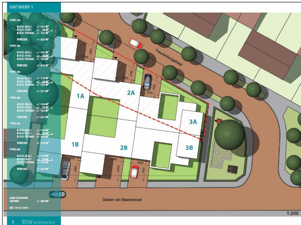
Figuur 3.1.1. (Voorlopige) schets van de voorgestane situatie. Bron: BenW Architecten.
