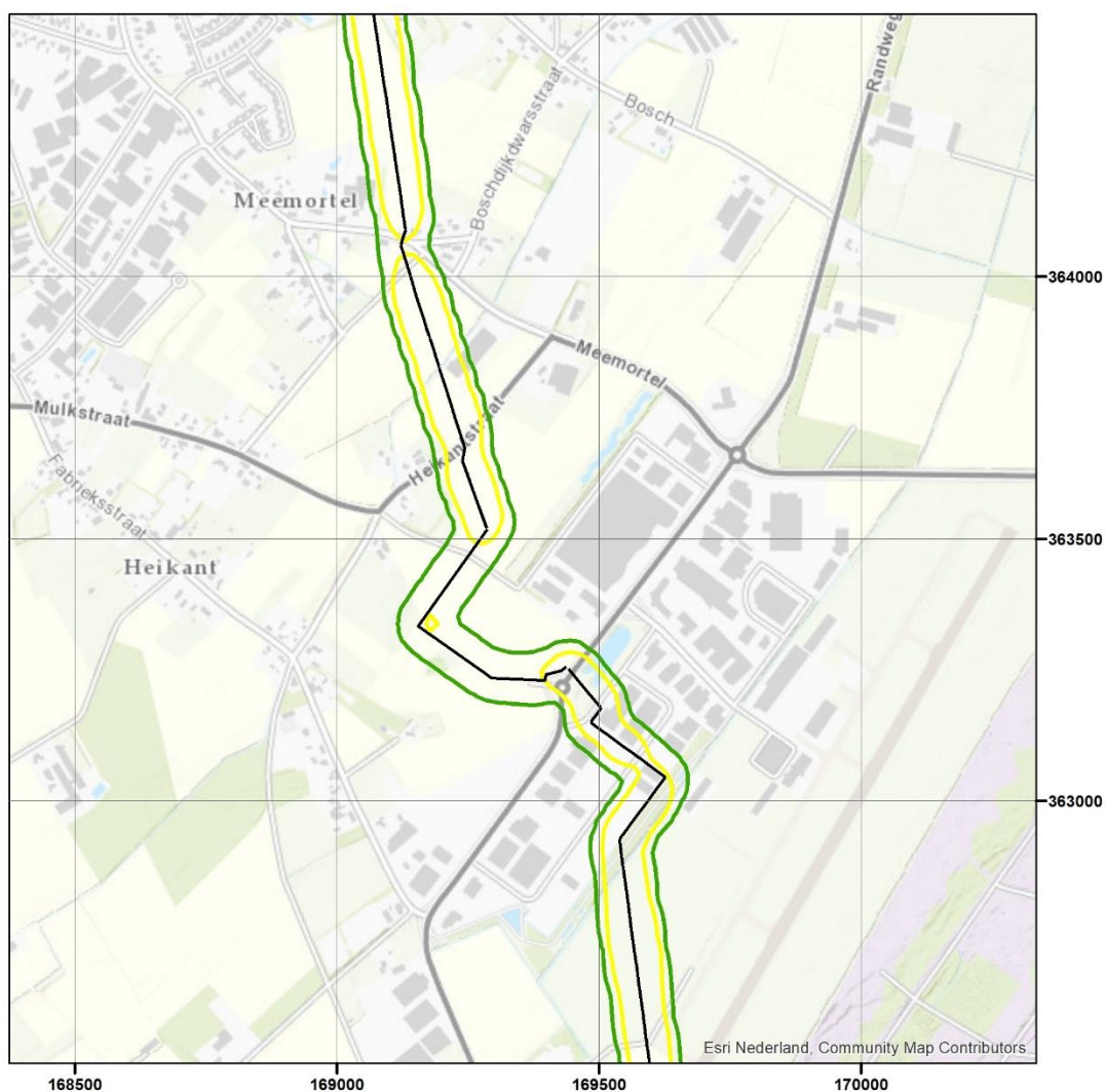
Figuur 3. PR-contouren aardgasleiding Z-532-05 toekomstige situatie
