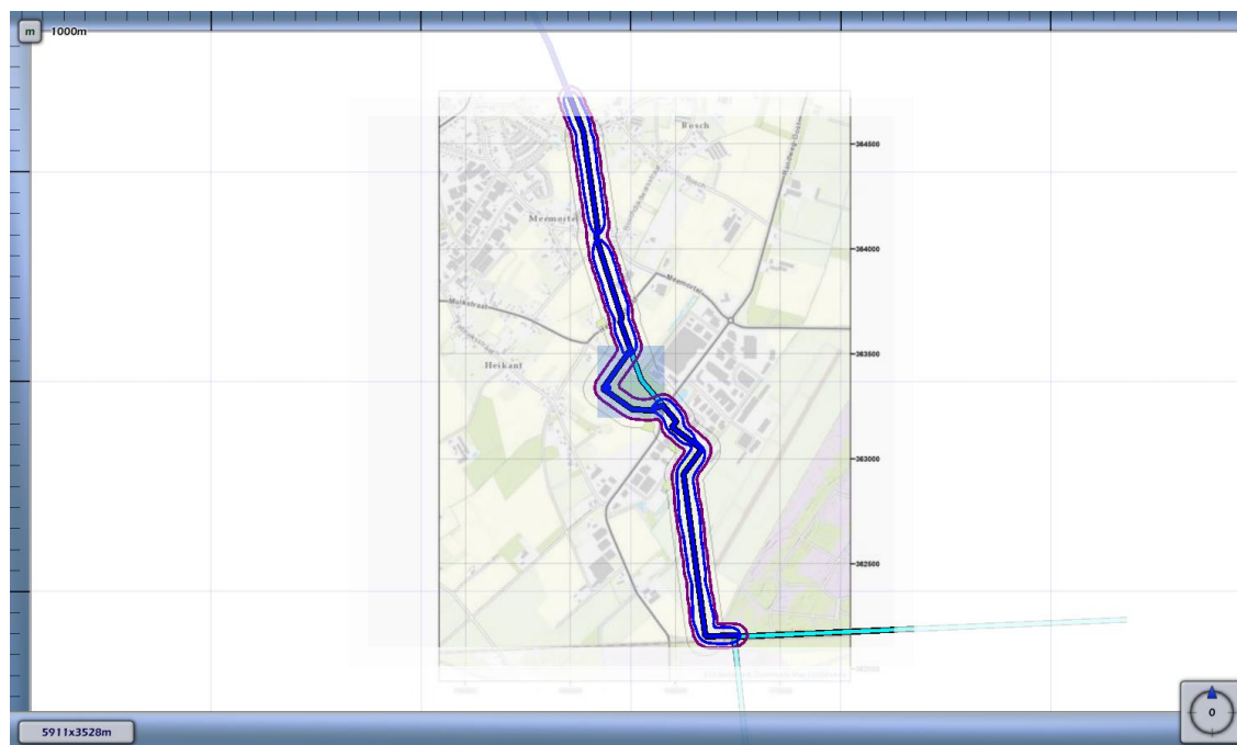
Figuur 3.2 Plaatsgebonden risico voor 5288_leiding-Z-532-05-deel-1_incl verl van N.V. Nederlandse Gasunie
