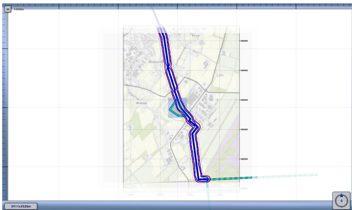
Figuur 3.1 Plaatsgebonden risico voor 5287_leiding-Z-532-05-deel-1_excl verl van N.V. Nederlandse Gasunie
