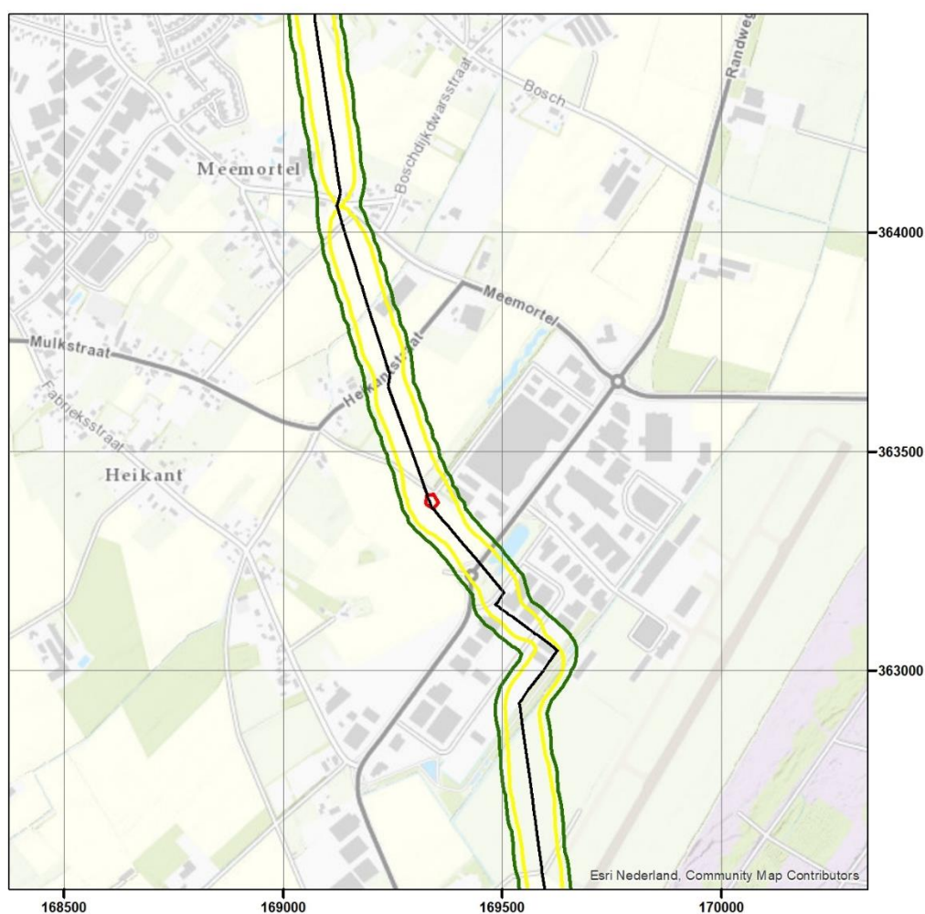
Figuur 2. PR-contouren aardgasleiding Z-532-05 huidige situatie
