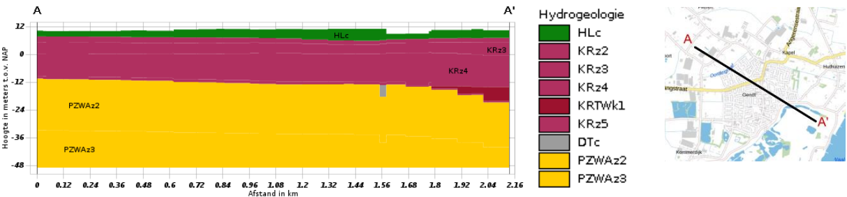
Figuur 1: Geohydrologisch model gebaseerd op REGIS II.1 (bron 3C)
