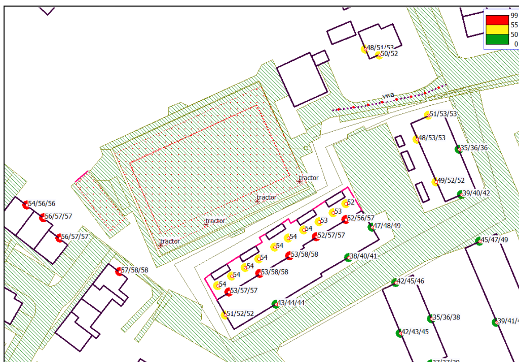
Figuur 6: Langtijdgemiddelde beoordelingsniveau doordeweekse dag, Activiteitenbesluit in dB(A) inclusief impulstoelag.
