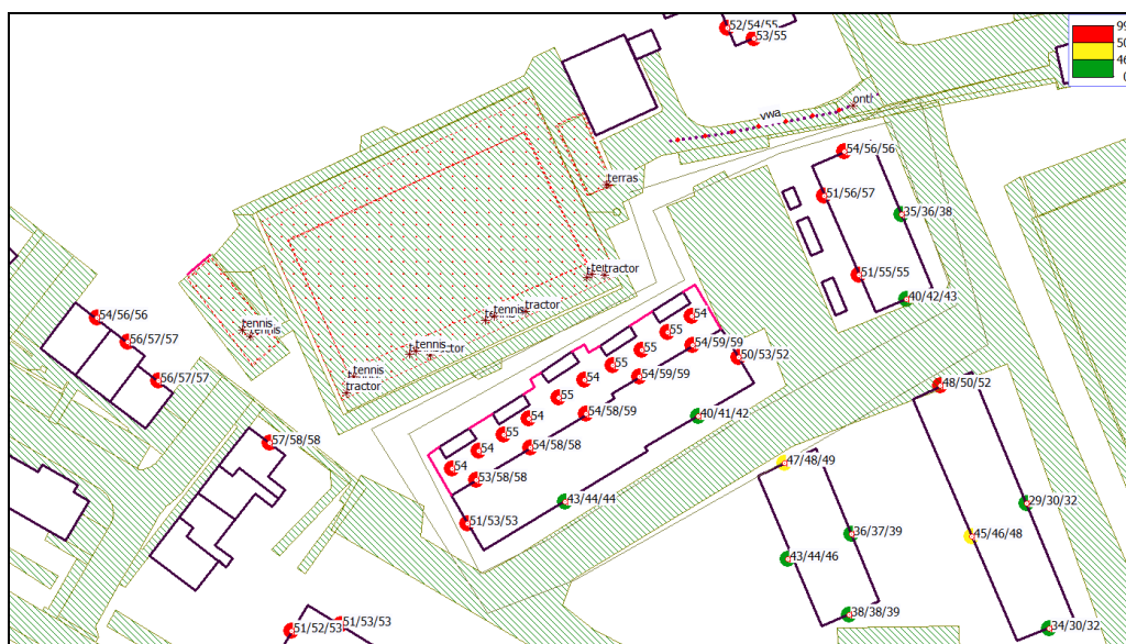
Figuur 7: Langtijdgemiddelde beoordelingsniveau doordeweekse dag, gemeentelijk beleid in dB(A), inclusief impuls toeslag.
