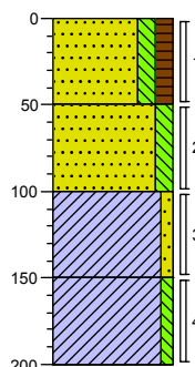
Boring/gat: 08
