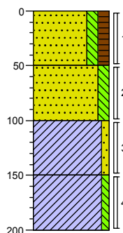
Boring/gat: 02
