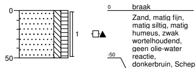
Boring: 10 boormeester J. Postma Sleuflengte [m]: 0,30 Sleufbreedte [m]: 0,30
