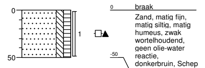
Boring: 09 boormeester J. Postma Sleuflengte [m]: 0,30 Sleufbreedte [m]: 0,30
