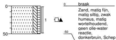
Boring: 07 boormeester J. Postma Sleuflengte [m]: 0,30 Sleufbreedte [m]: 0,30
