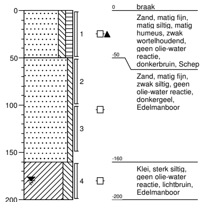
Boring: 11 boormeester J. Postma Sleuflengte [m]: 0,30 Sleufbreedte [m]: 0,30
