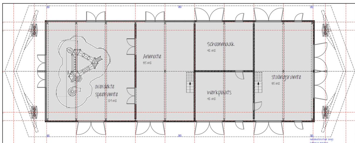
Afbeelding 4 Plattegrond begane grond voorzieningengebouw (Bron: Architectenburo van ruth bv)
