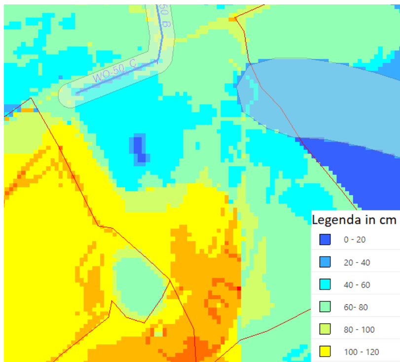
Figuur 2 Kaartbeeld bestaande grondwaterstand rond het plangebied.
