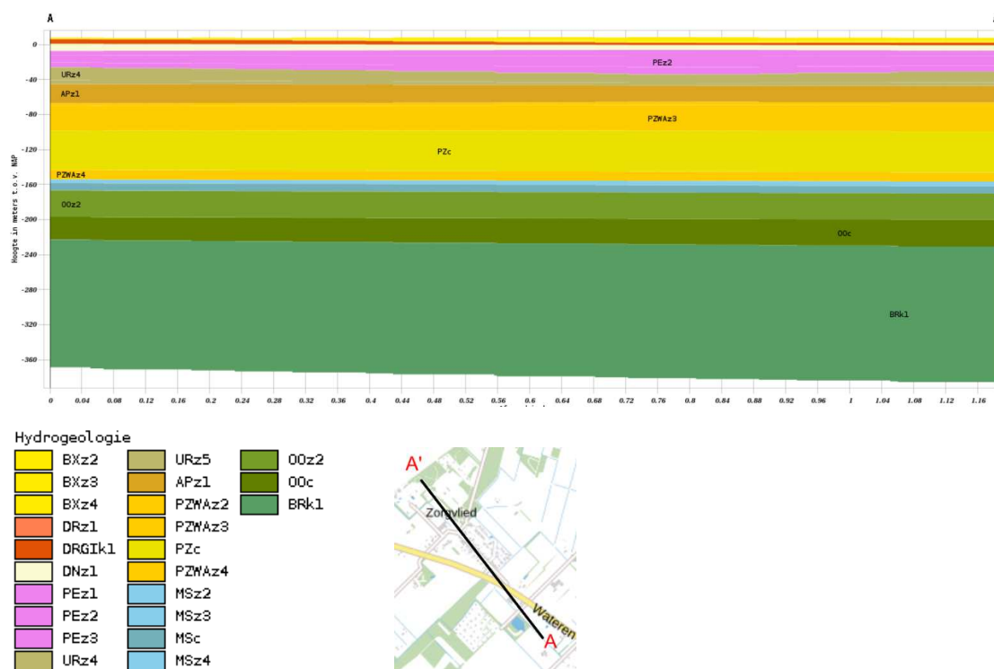
figuur 1: de geohydrologische opbouw
