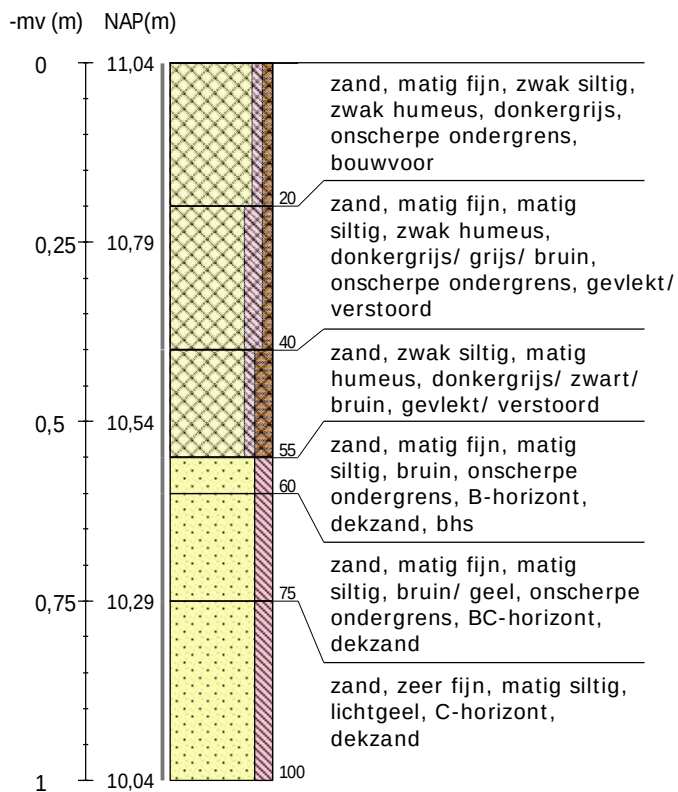
Boring 1 RD-coördinaten: 223702/543822
