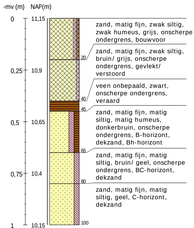
Boring 11 RD-coördinaten: 223640/543837
