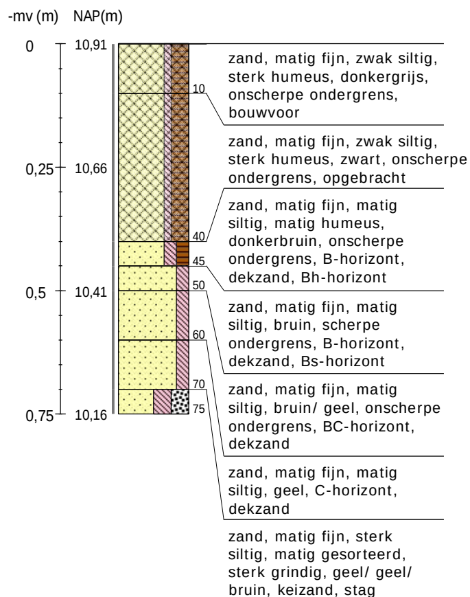
Boring 8 RD-coördinaten: 223645/543726
