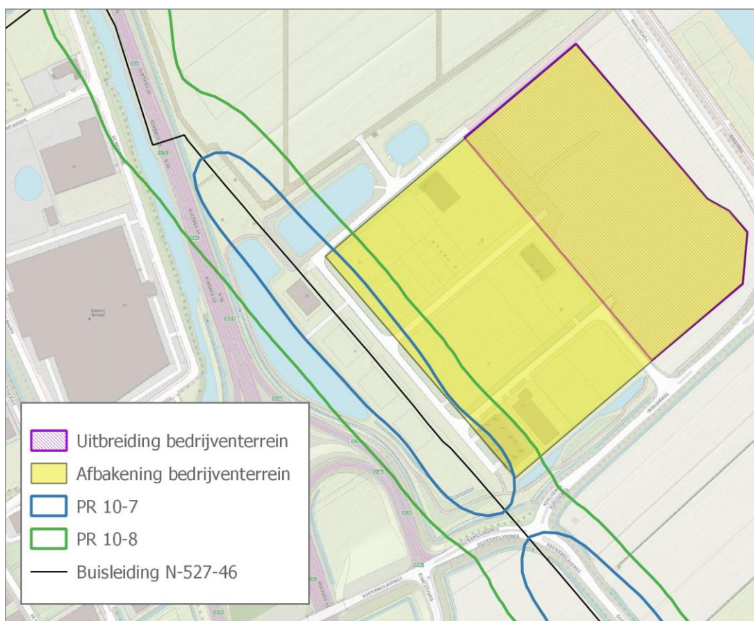
Figuur 5. PR-contouren aardgasleiding N-527-46
