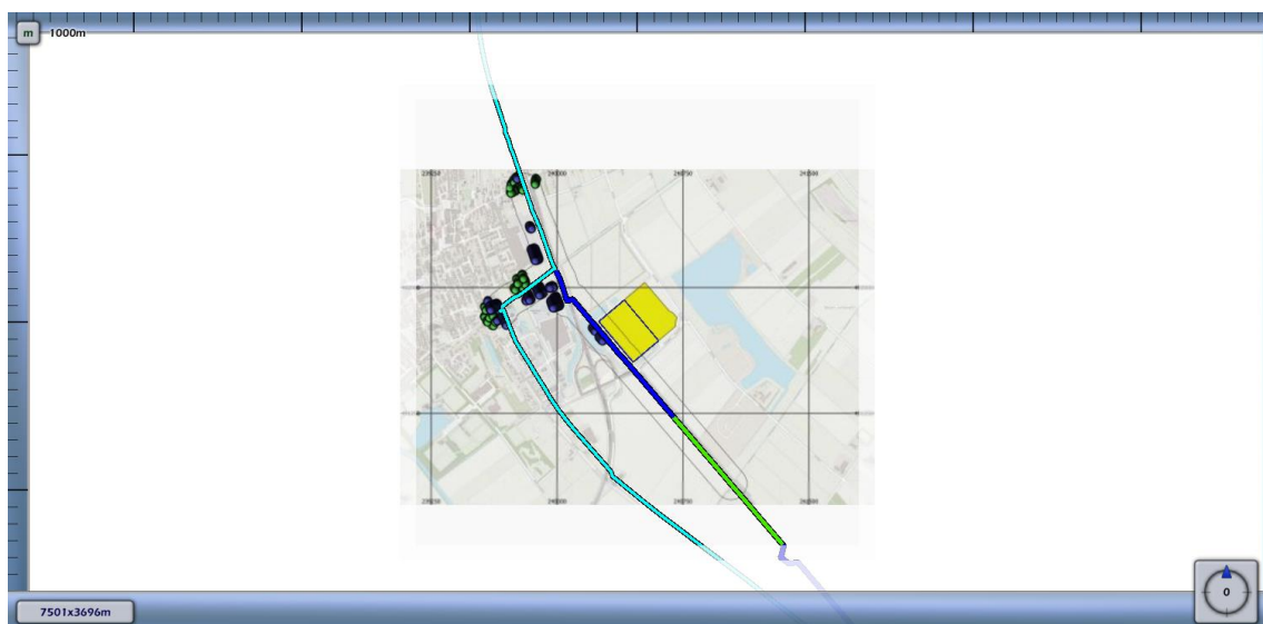
Figuur 4.2 Kilometer leiding behorende bij de maximale overschrijding van de FN-curve voor 8062_leiding-N-527-46-deel-1 van N.V. Nederlandse Gasunie
