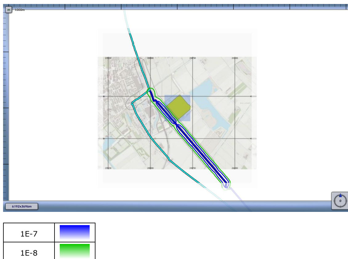
Figuur 3.1 Plaatsgebonden risico voor 8062_leiding-N-527-46-deel-1 van N.V. Nederlandse Gasunie
