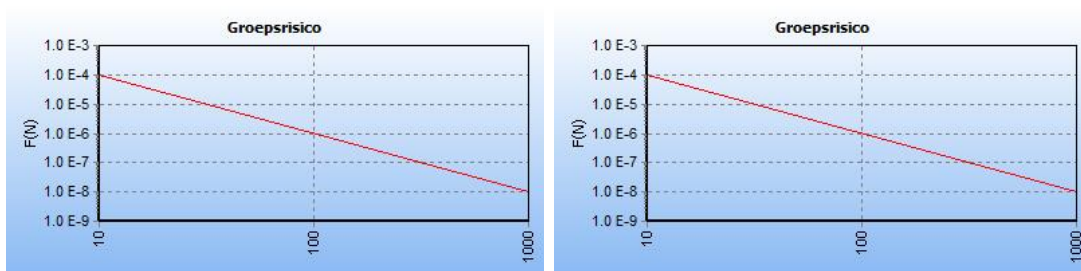
Figuur 6 Groepsrisico N-527-46, huidig (links) en toekomstig (rechts)
