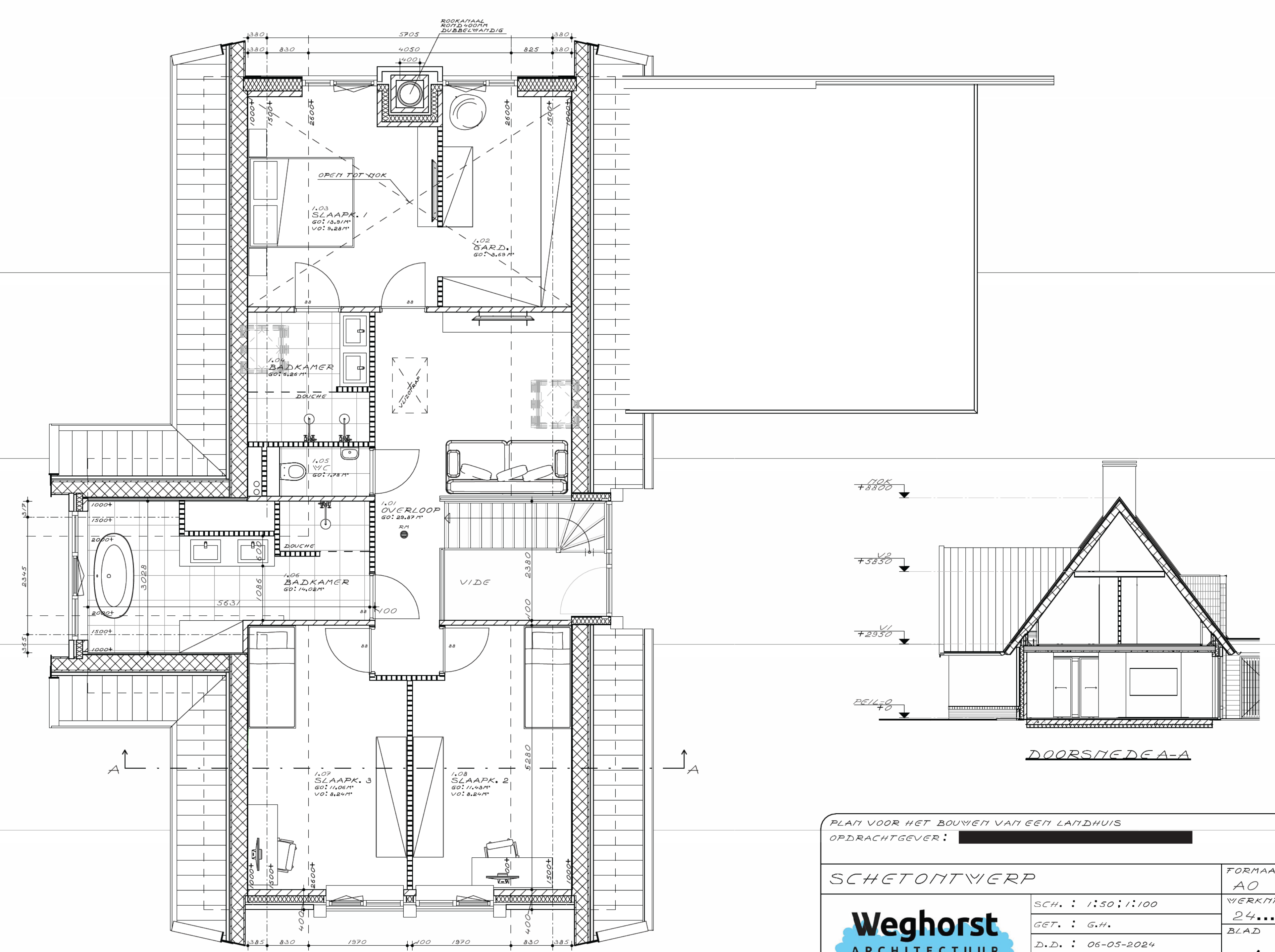
1e VERDIEPING
