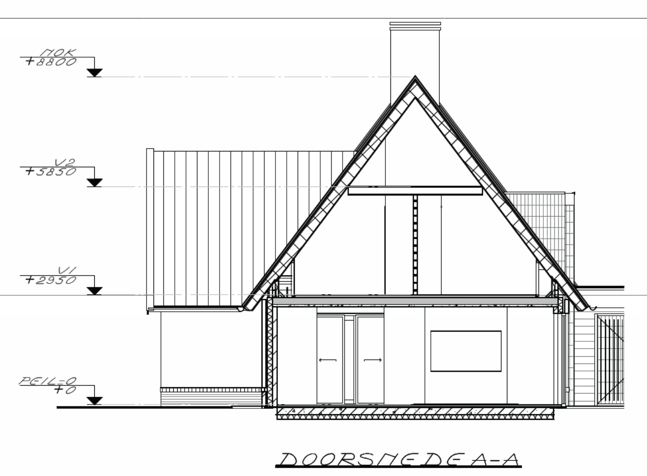
DOORSNEDENA-A
