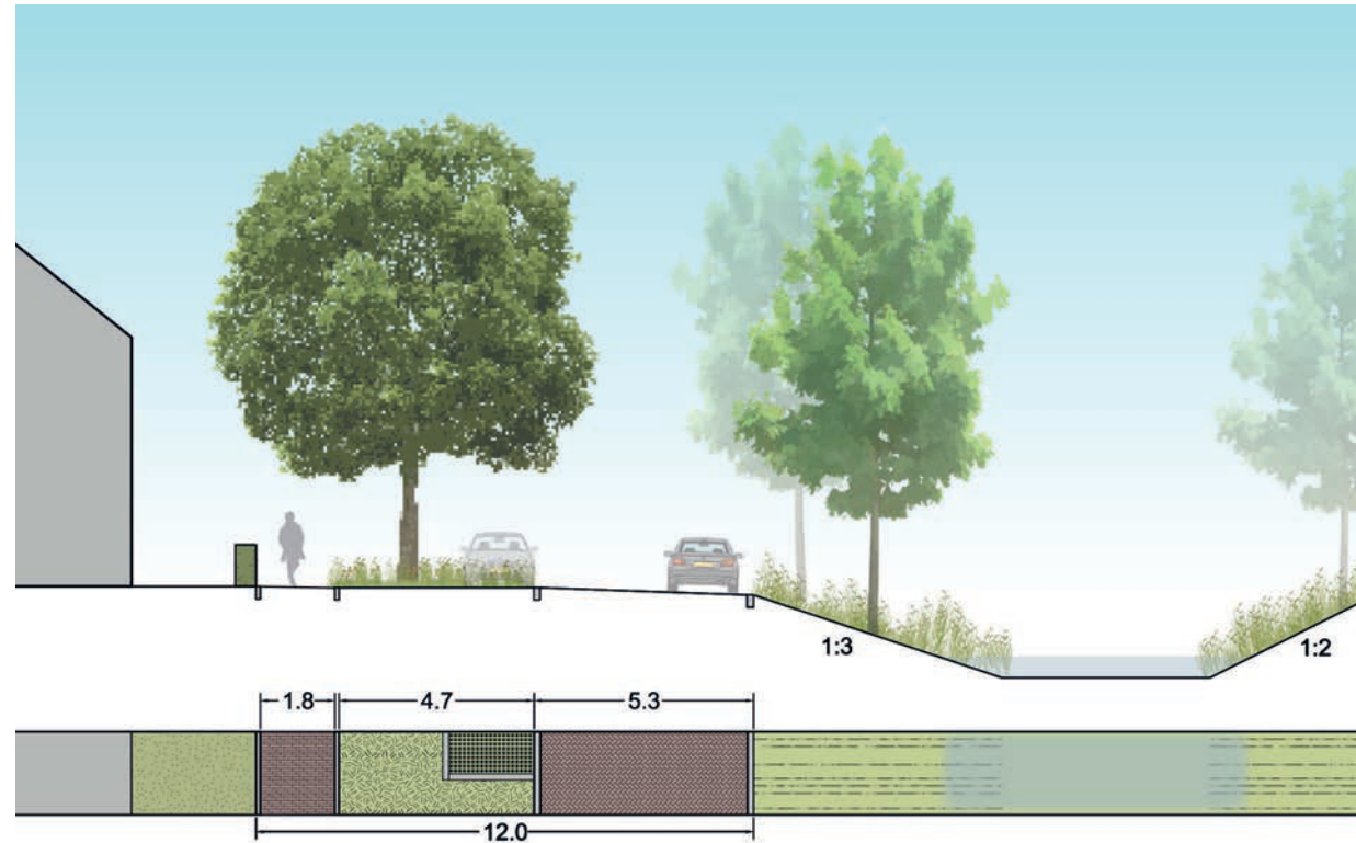
Principe profiel dorpsring met watergang
