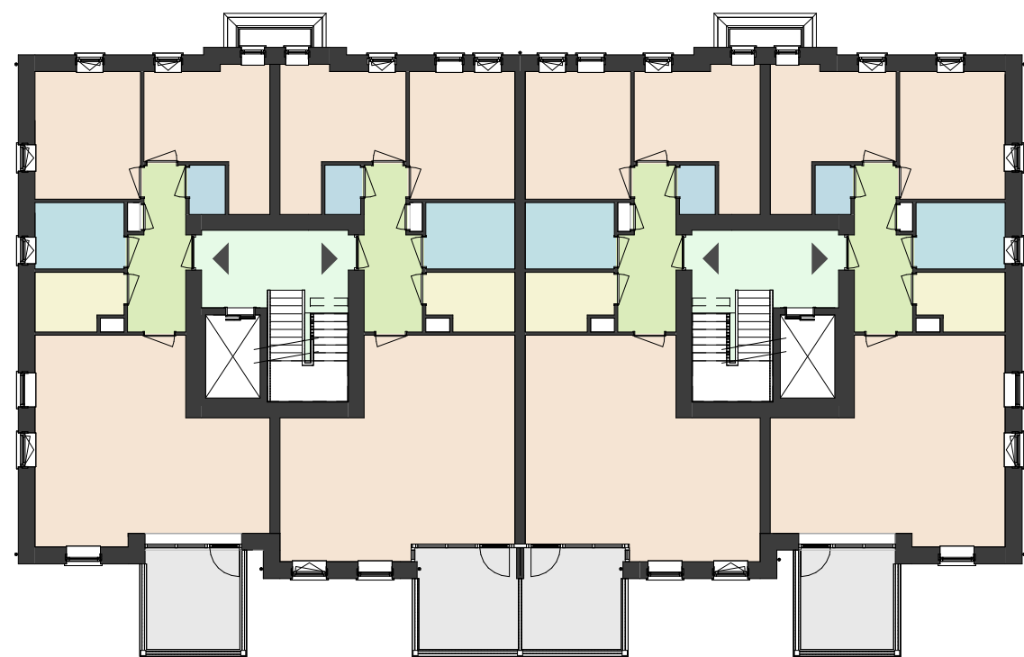
hoek-appartement 3 - kamer appartement BVO 99 m² GO 81 m² buitenruimte 10,0 m² tussen-appartement 3 - kamer appartement BVO 96 m² GO 84 m² buitenruimte 10,0 m²
