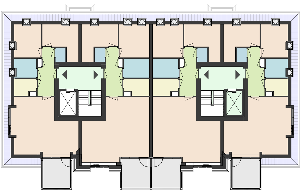
hoek-appartement 3 - kamer appartement BVO 97 m² GO 73 m² buitenruimte 10,0 m² tussen-appartement 3 - kamer appartement BVO 95 m² GO 81 m² buitenruimte 10,0 m²
