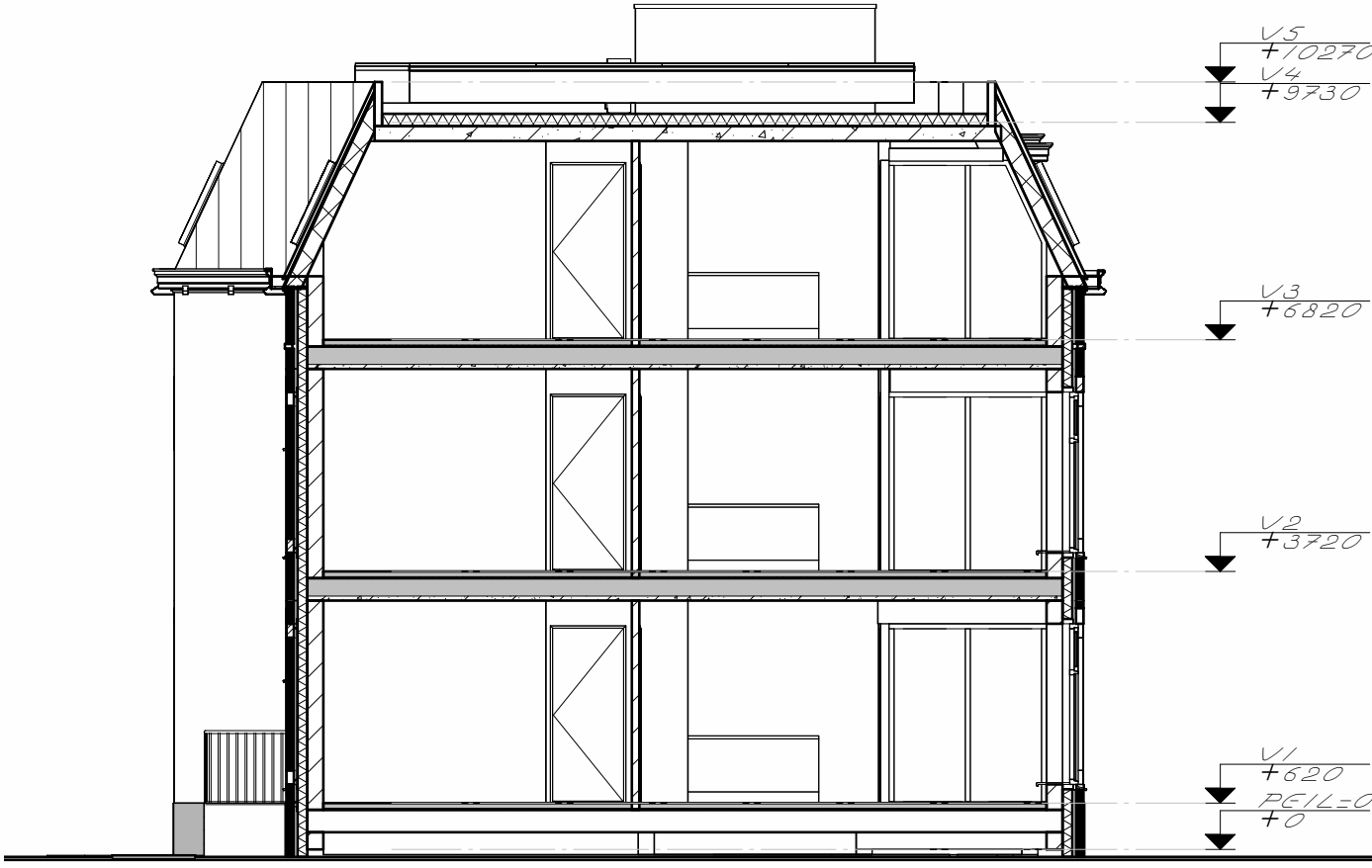
DOORSNEDEN B-B
