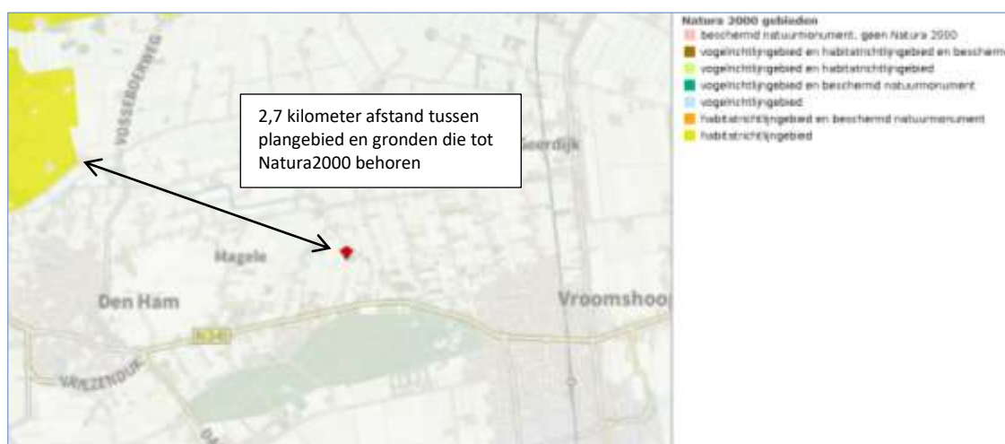
Ligging van Natura2000-gebied in de omgeving van deelgebied Wittenbrink. De ligging van het plangebied wordt met de rode marker aangeduid. Gronden die tot Natura2000 behoren worden met de okergele kleur aangeduid (bron: PDOK.nl).
