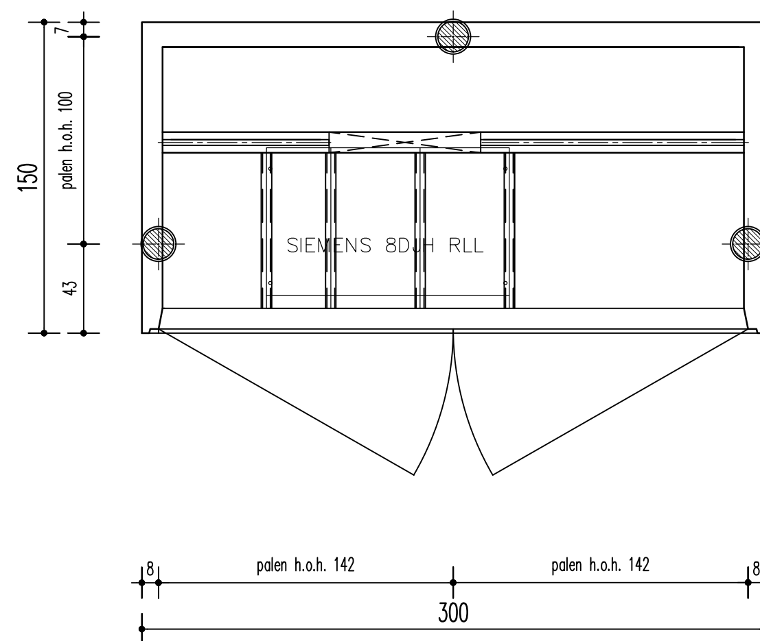
Installatie plattegrond en palenplan
