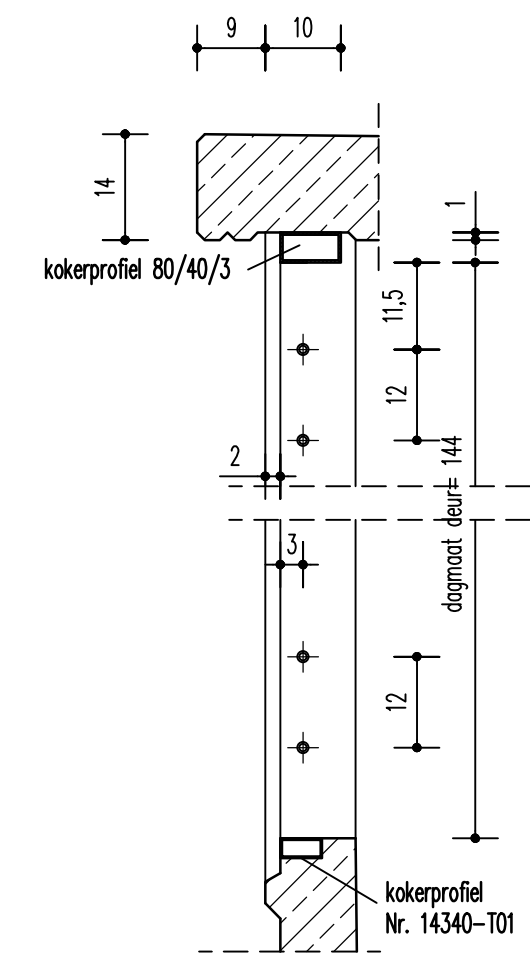
Detail 1:10 Alu-deur
