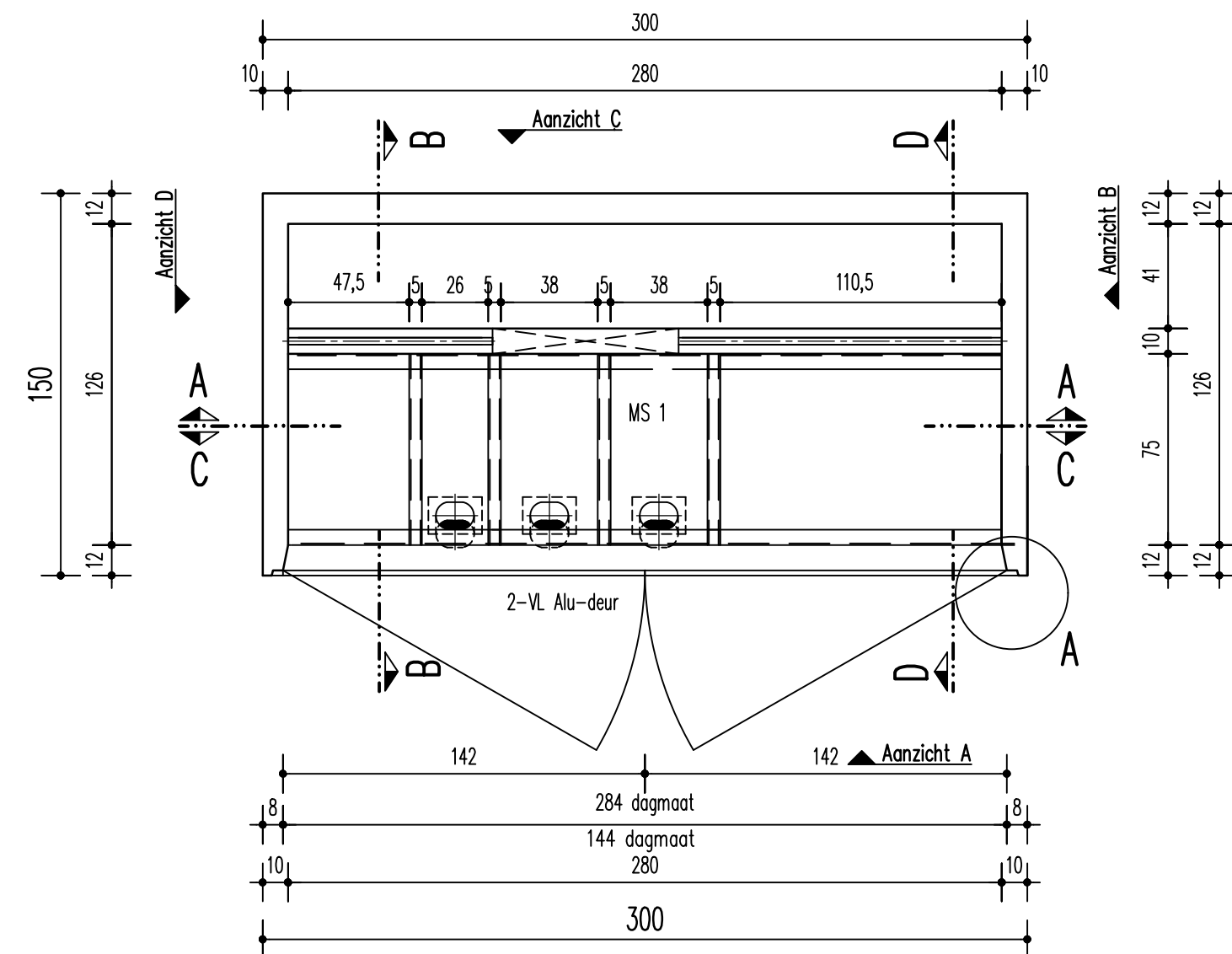
Plattegrond
