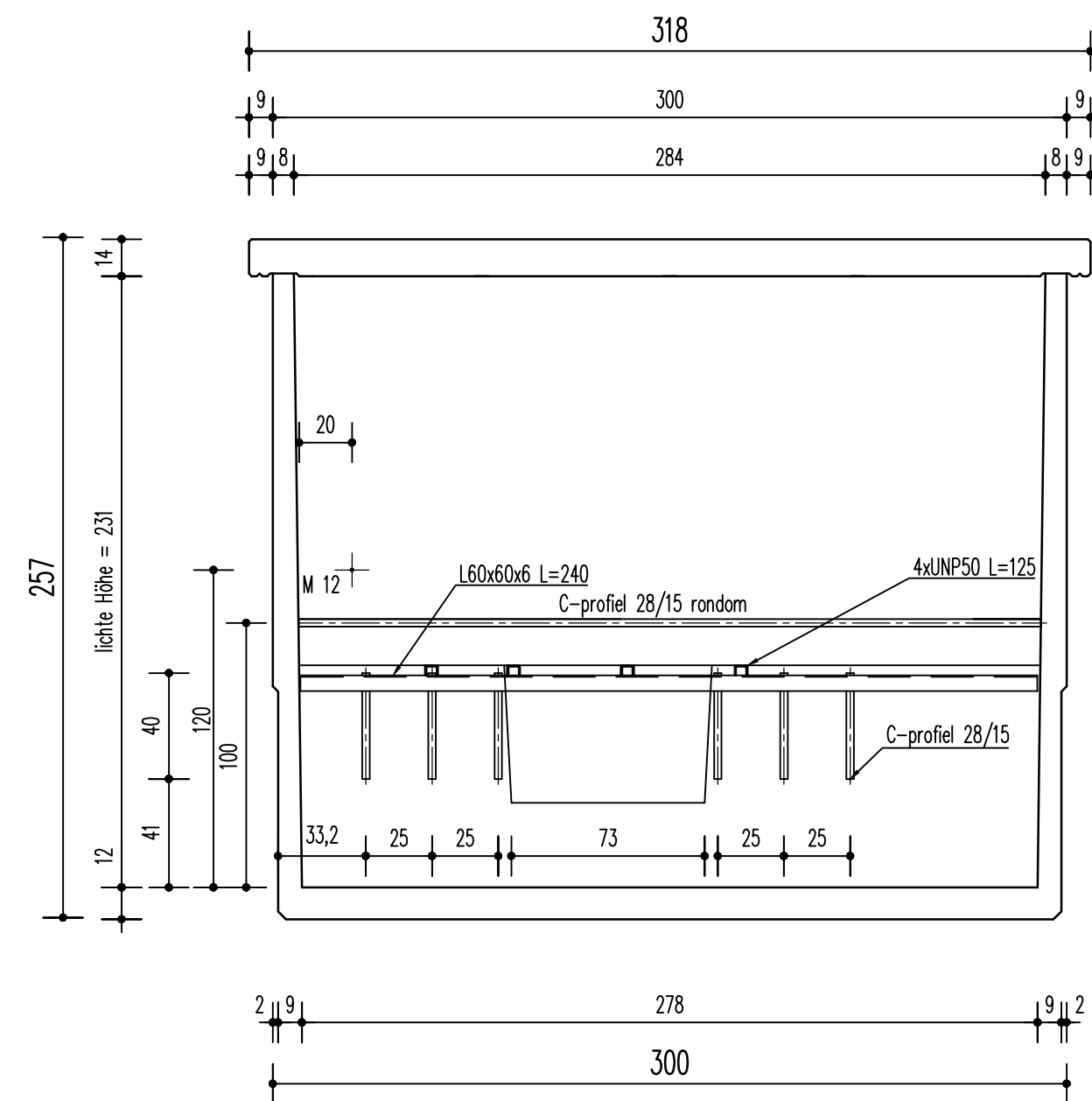
Doorsnede A-A
