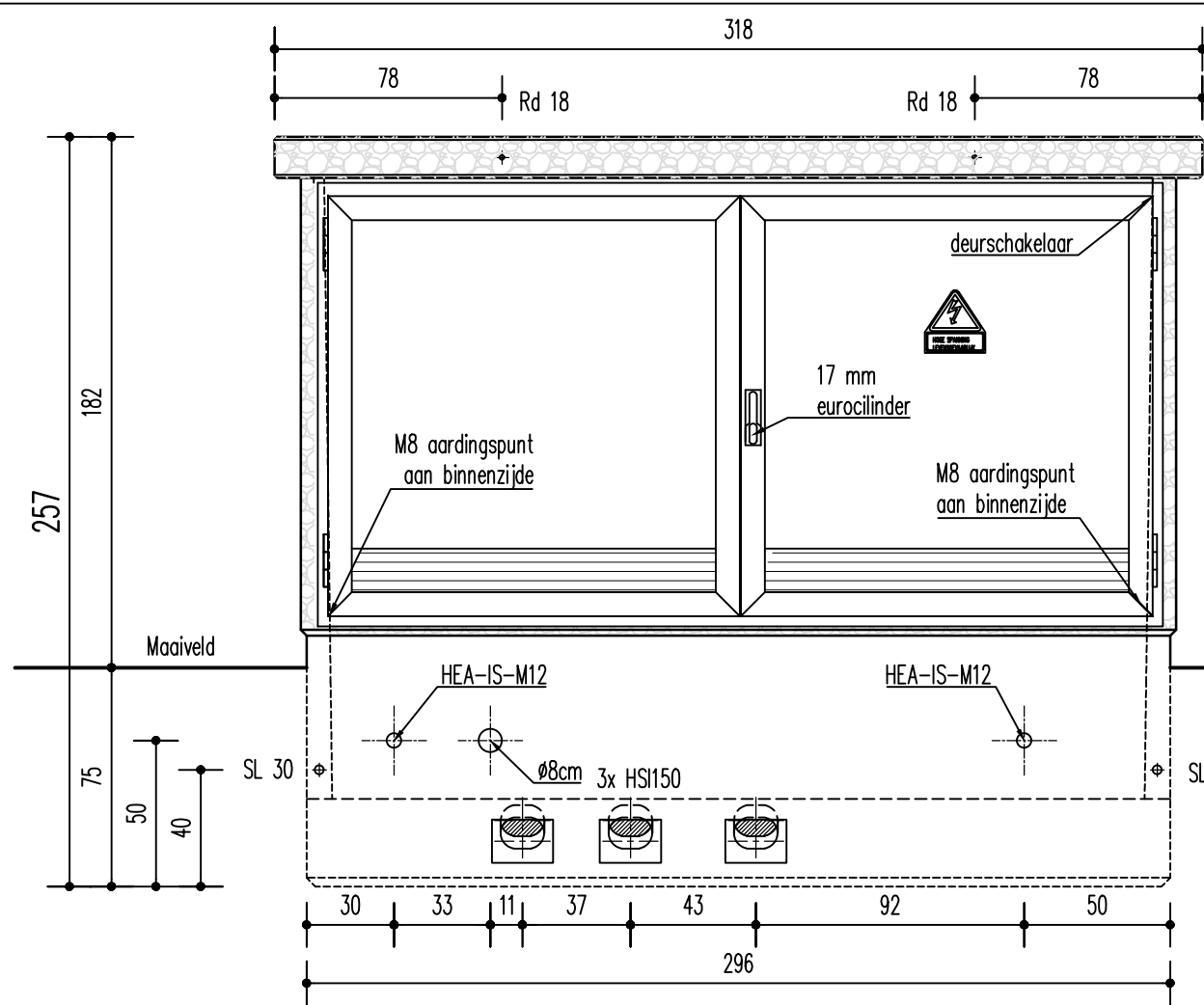
Aanzicht A
