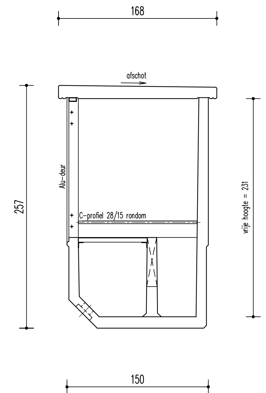
Doorsnede D-D
