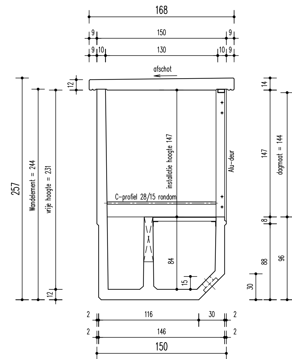
Doorsnede B-B
