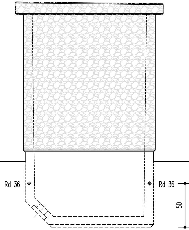
Aanzicht B
