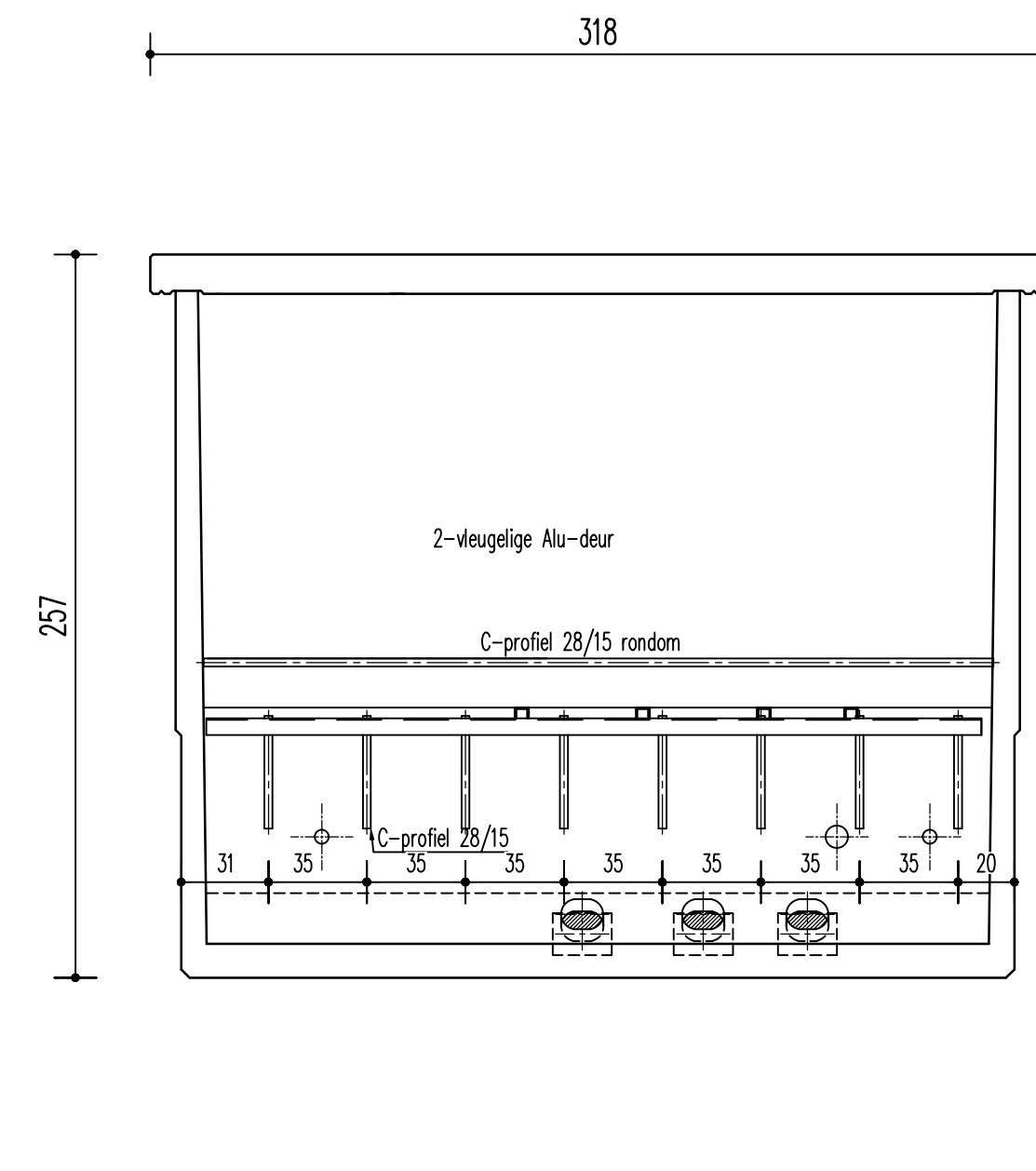
Doorsnede C-C
