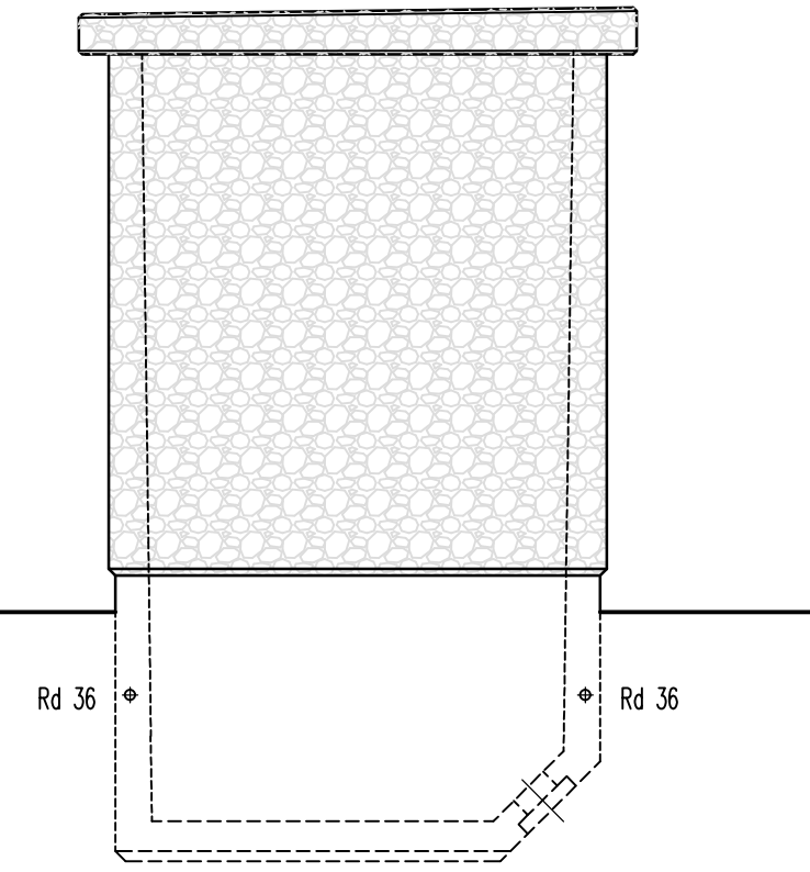
Aanzicht D
