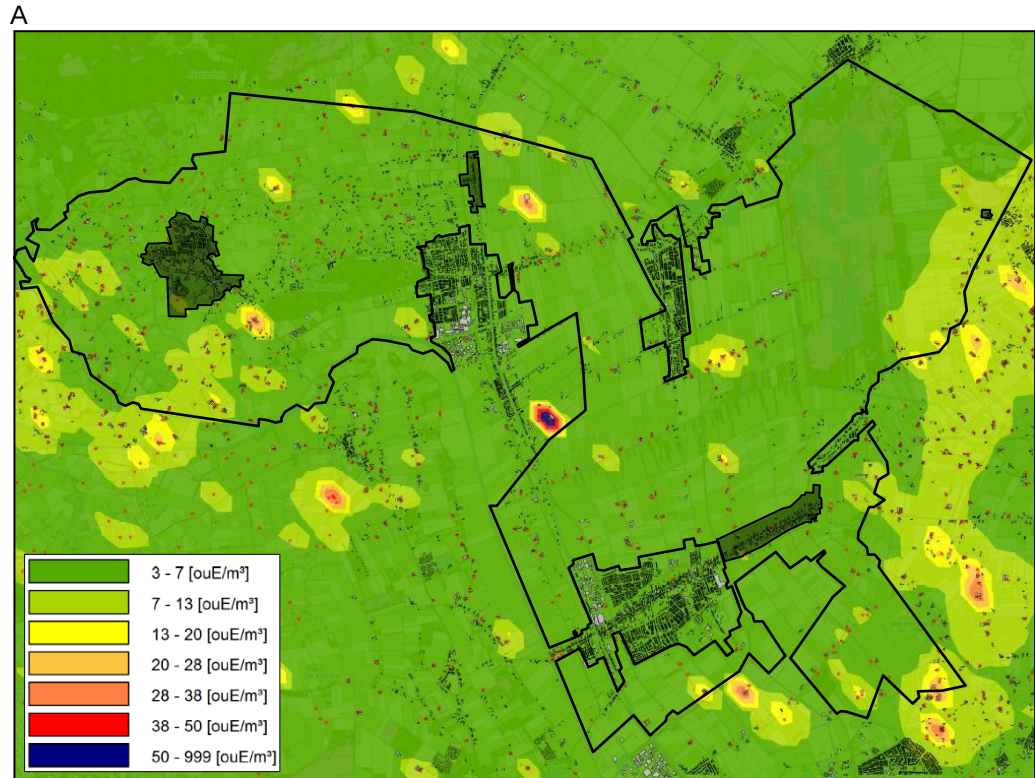
Figuur: achtergrondbelasting geur in de referentiesituatie (bron: Windmill)
