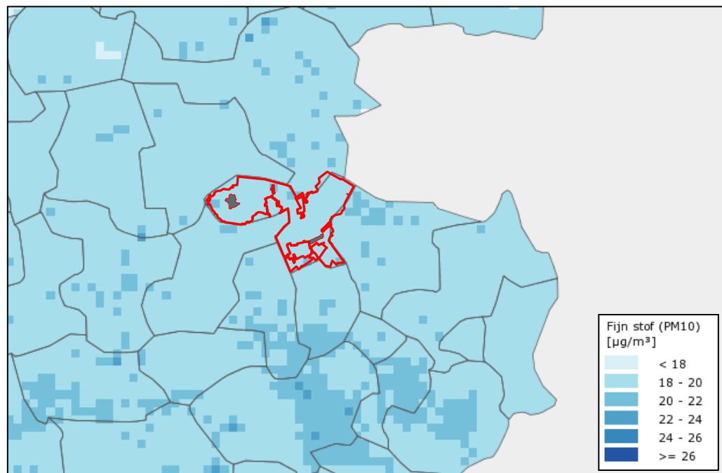
Fijn stofconcentratie PM 10 Twenterand 2020 (bron: GCN kaarten Nederland)
