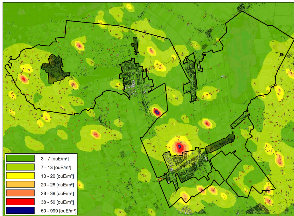
Figuur: achtergrondbelasting geur in de maximalisatie van het voornemen (bron: Windmill)
