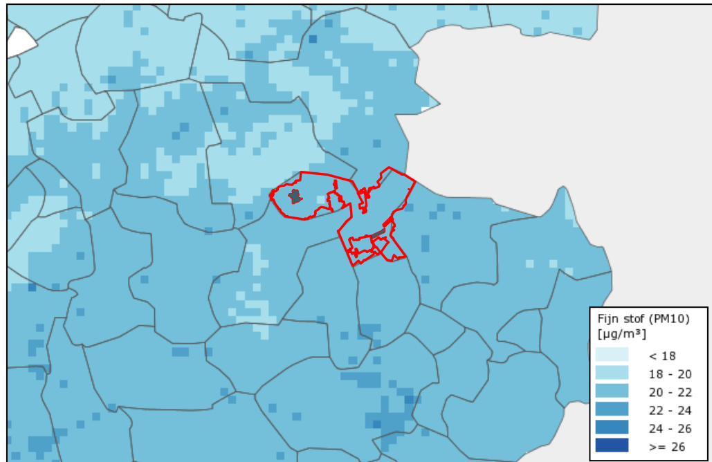
Fijn stofconcentratie PM 10 Twenterand 2015 (bron: GCN kaarten Nederland)
