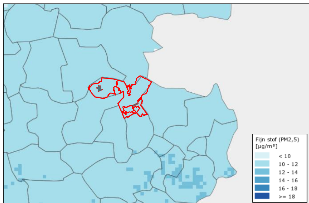
Fijn stofconcentratie PM 2,5 Twenterand 2020 (bron: GCN kaarten Nederland)
