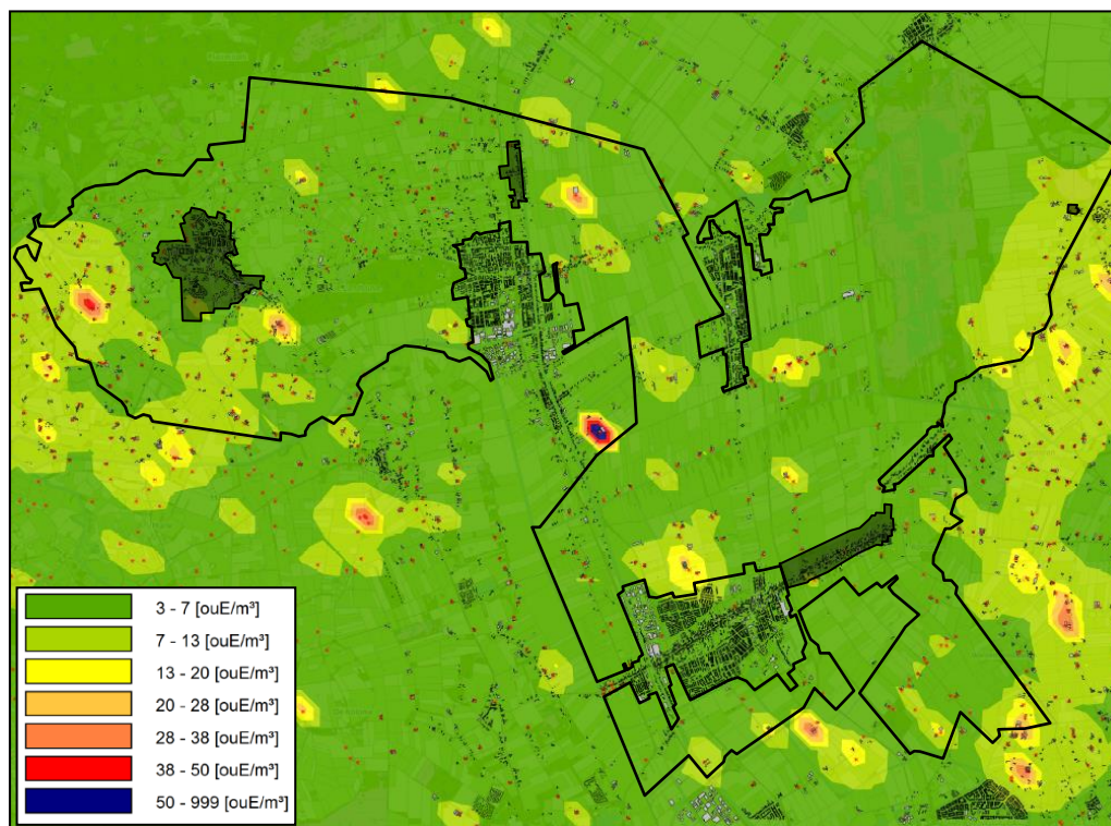
Figuur: achtergrondbelasting geur in de maximalisatie van het alternatief (bron: Windmill)
