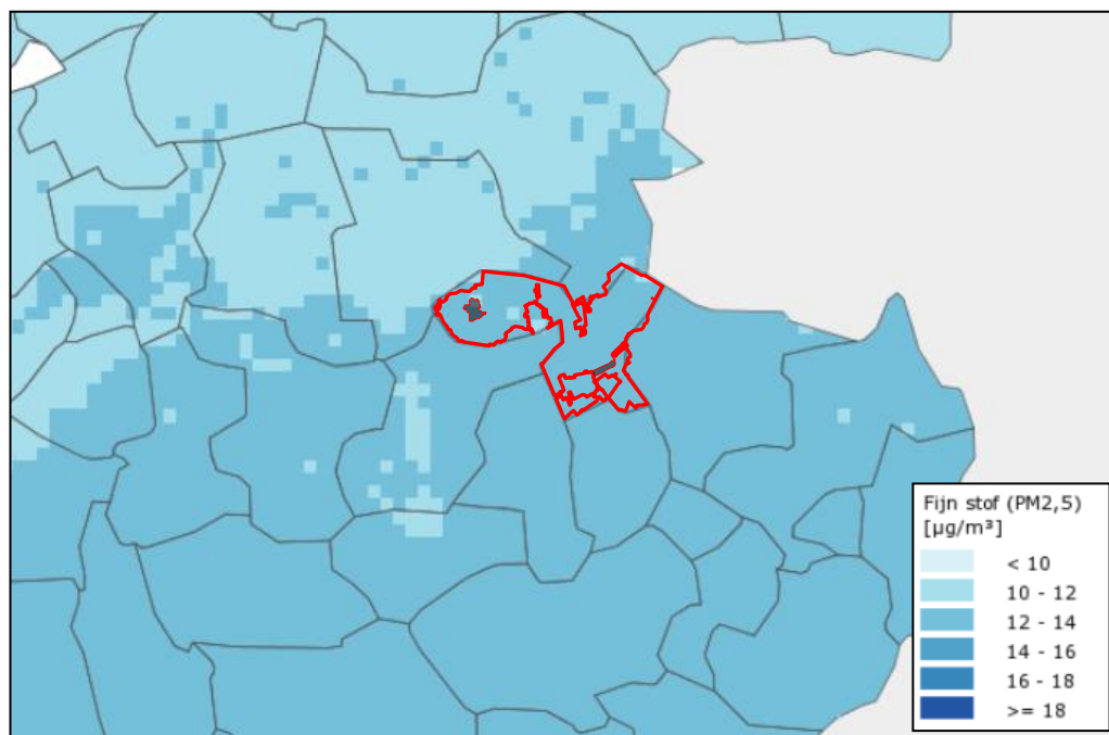
Fijn stofconcentratie PM 2,5 Twenterand 2015 (bron: GCN kaarten Nederland)
