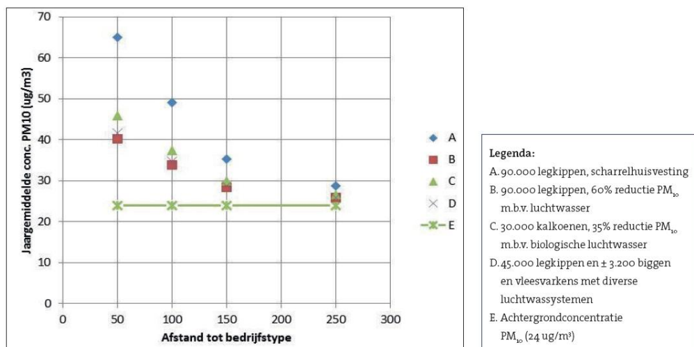
Berekende concentraties PM_{10} in relatie tot de afstand tot de veehouderij 19
