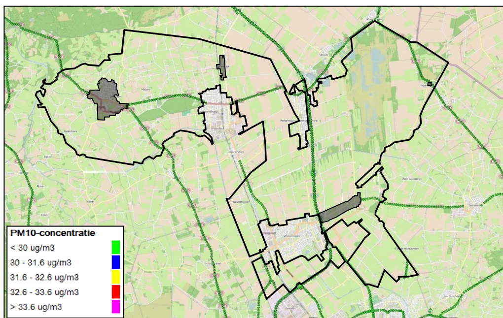
Weergave van de fijn stofconcentratie rond wegen in 2015 (bron: monitoringstool)
