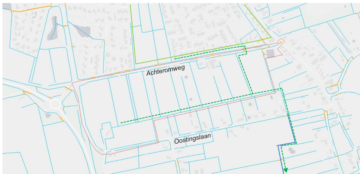
Figuur 3 Watersysteem in het plangebied (binnen rode lijn) in de huidige situatie. Sloten (lichtblauwe lijnen) binnen het plangebied zijn in particulier beheer. Hoofdwatervangsten (donkerblauwe lijn) zijn in het beheer van het waterschap. Met een groene stippellijn is de hoofdafvoerstructuur aangegeven.
