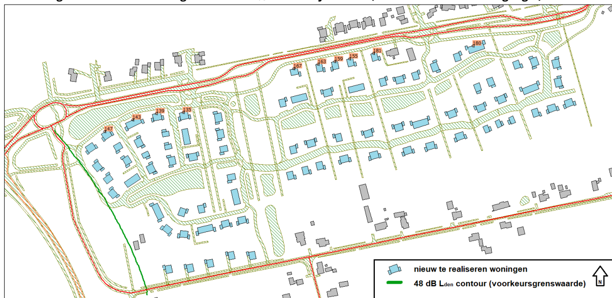
Afbeelding 3.3: Bunnerveenseweg N386 48 dB L den contour jaar 2031 (incl. 2 dB aftrek art. 110g Wgh.)
