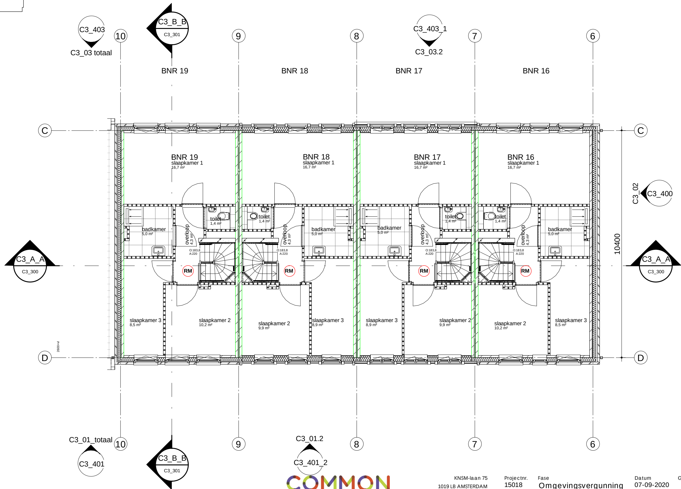
02 tweede verdieping - C3_2
