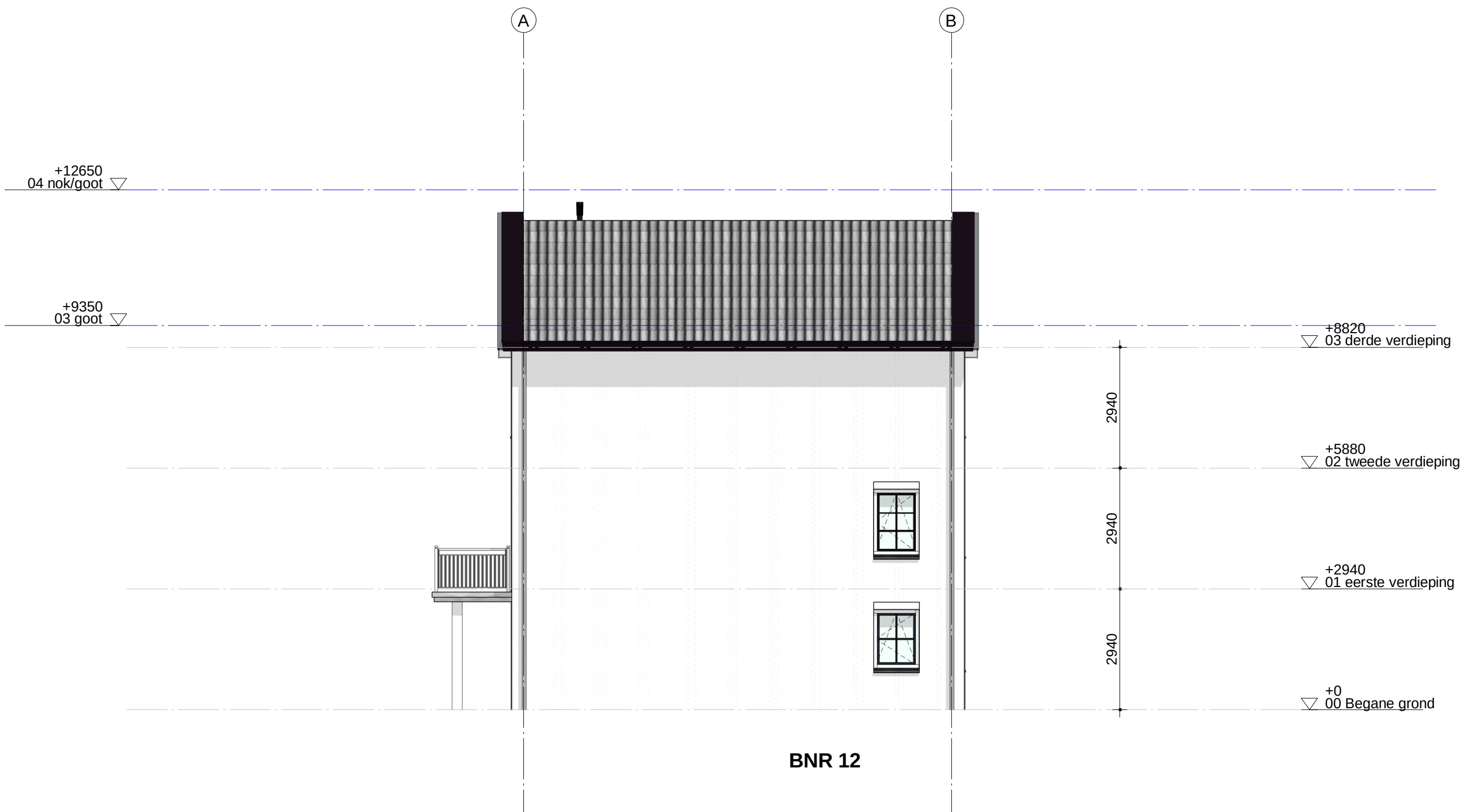
C2_04_Oostgevel
