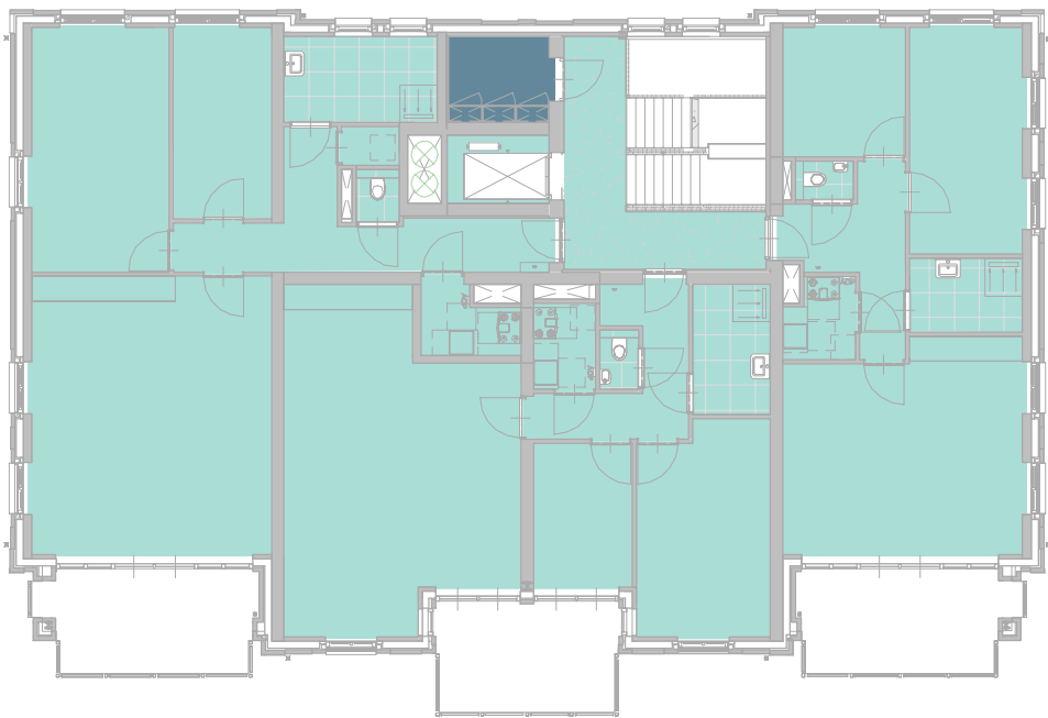
Eerste verdieping
