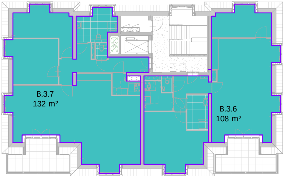
03 derde verdieping
