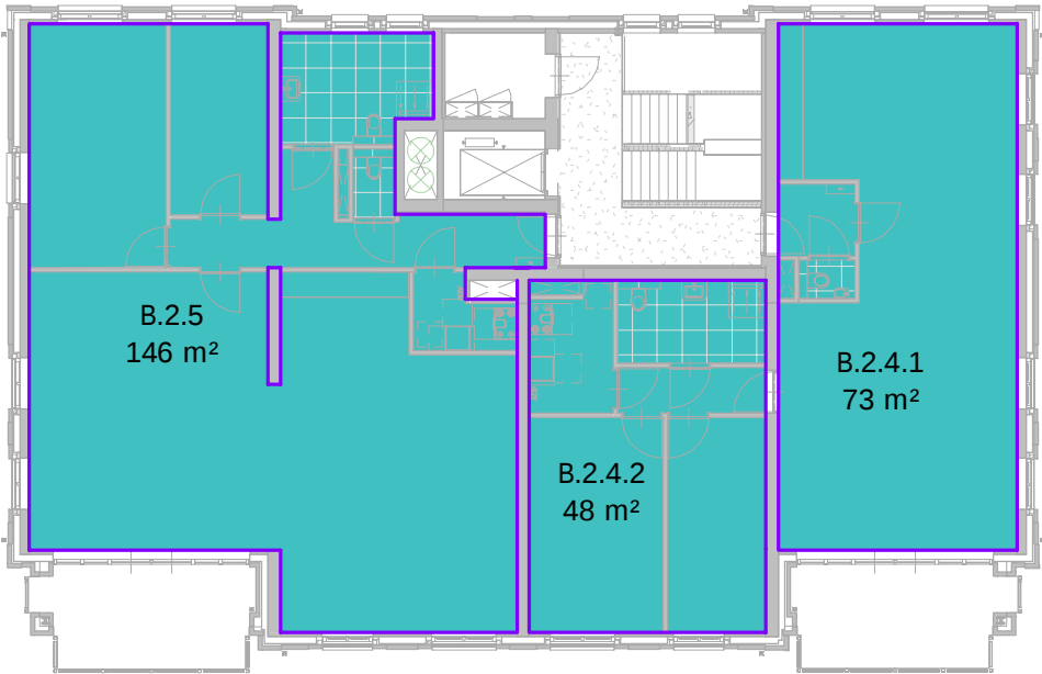
02 tweede verdieping
