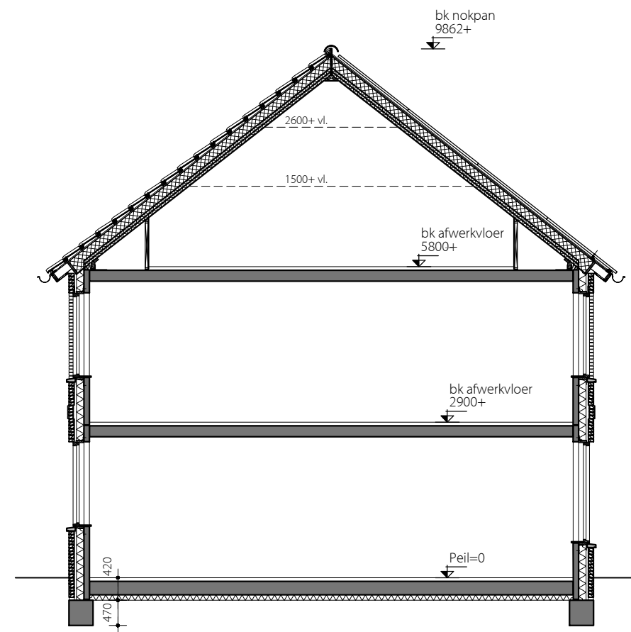
Doorsnede laagbouw
