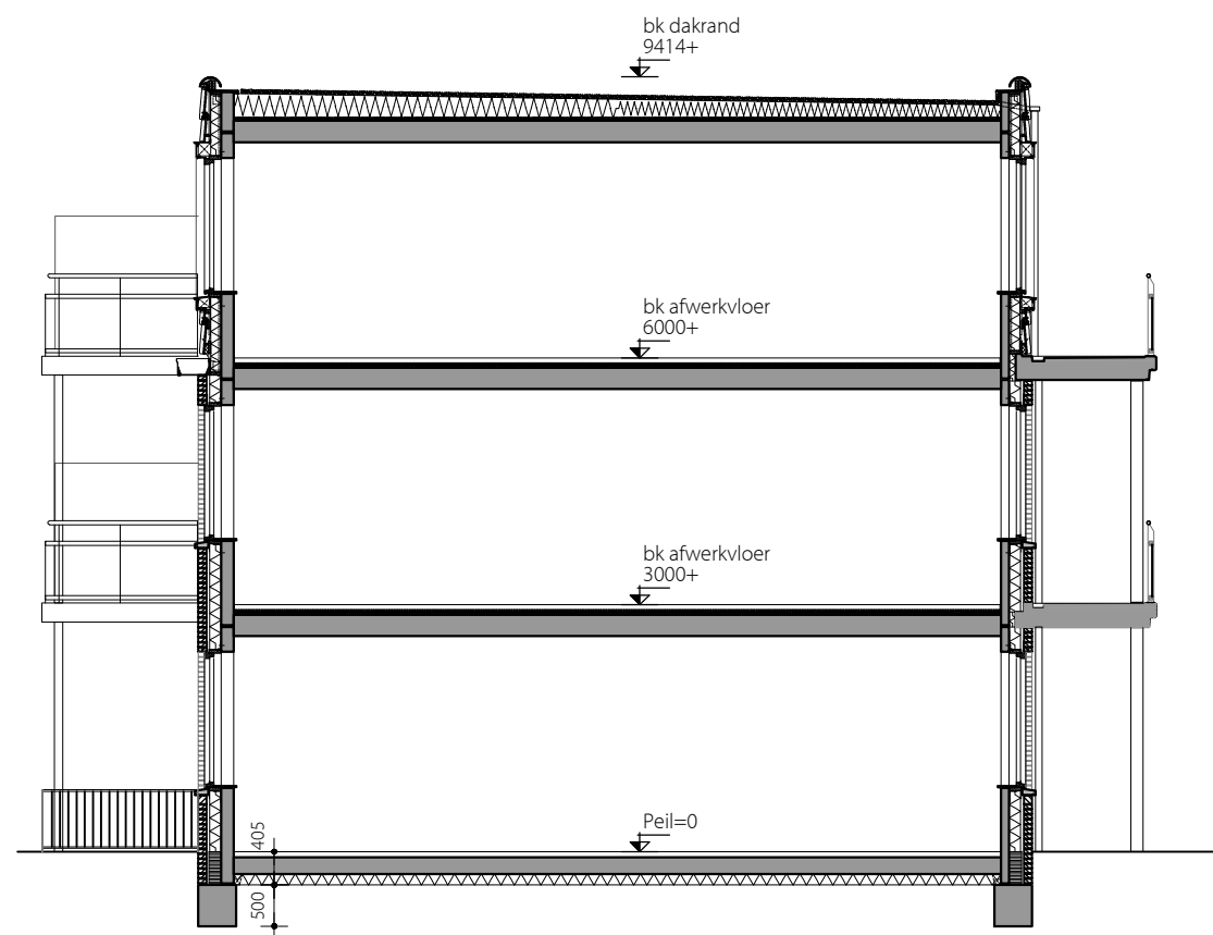
Doorsnede appartementen
