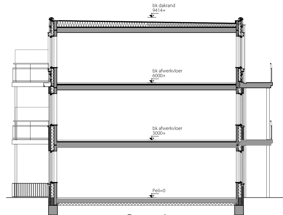
Doorsnede
