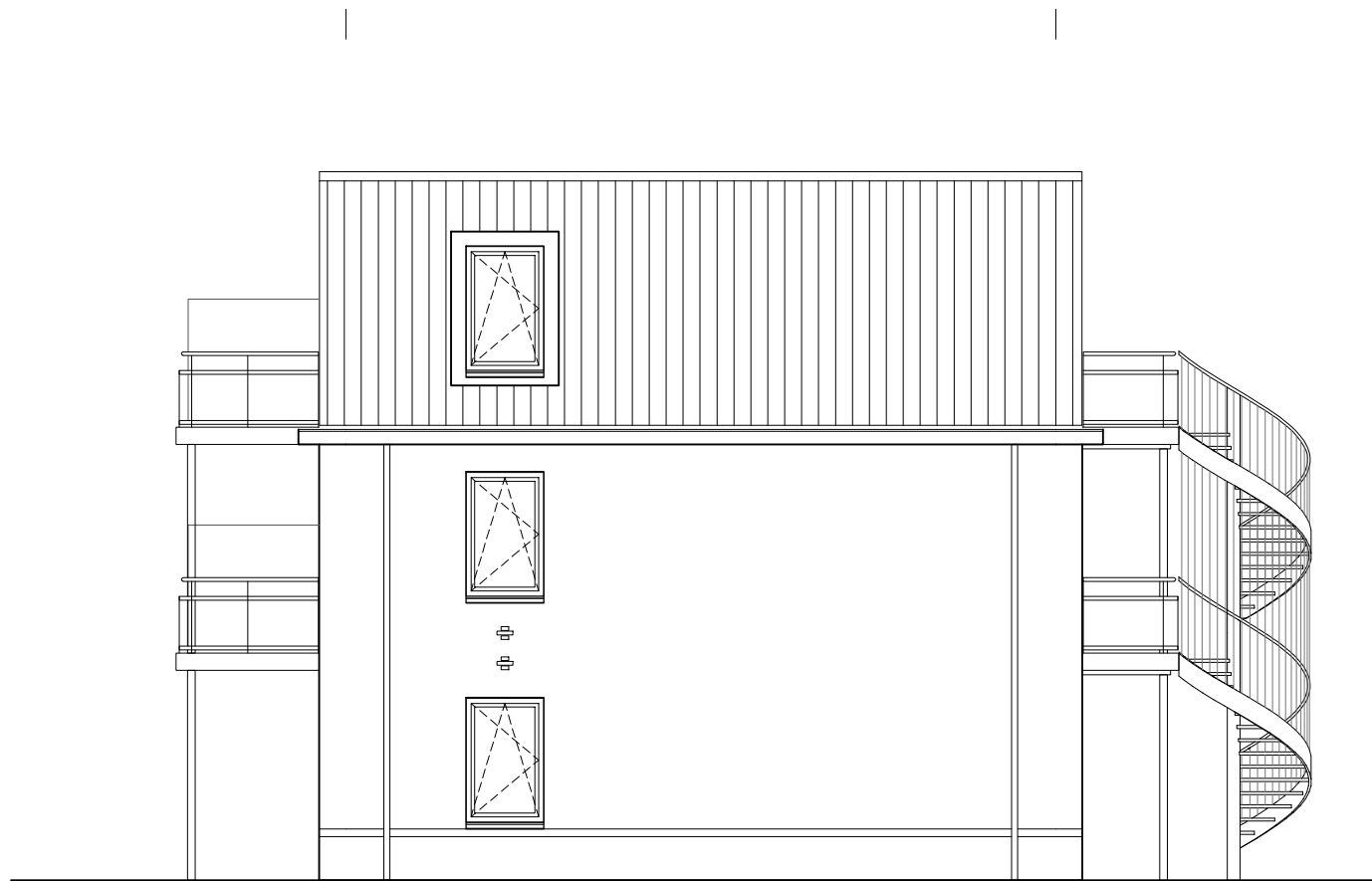
Rechter Zijgevel
