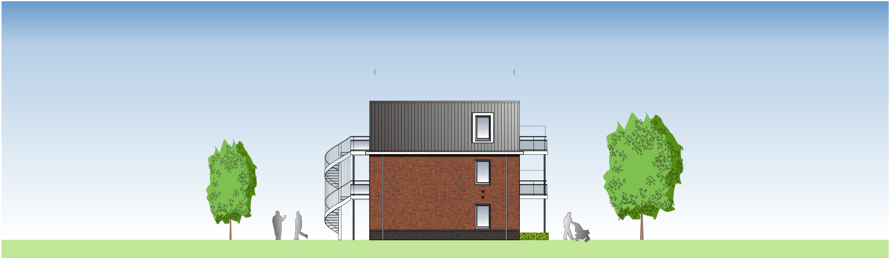
Linker Zijgevel
