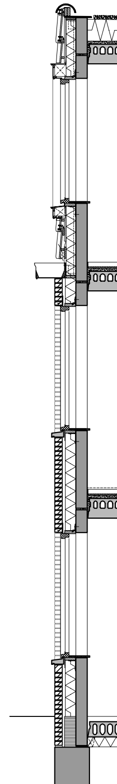
Fragment gevel
