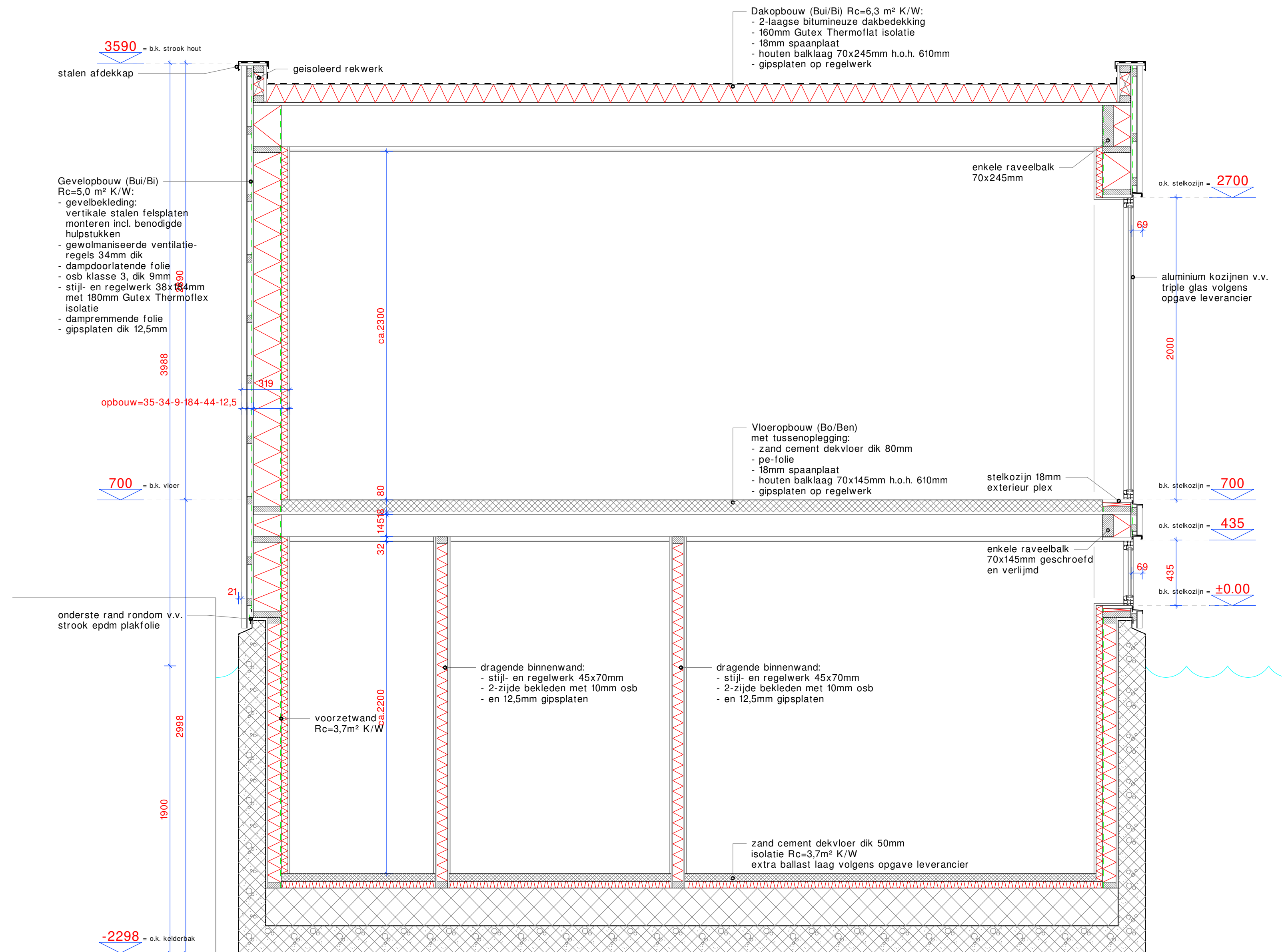
Doorsnede A-A
