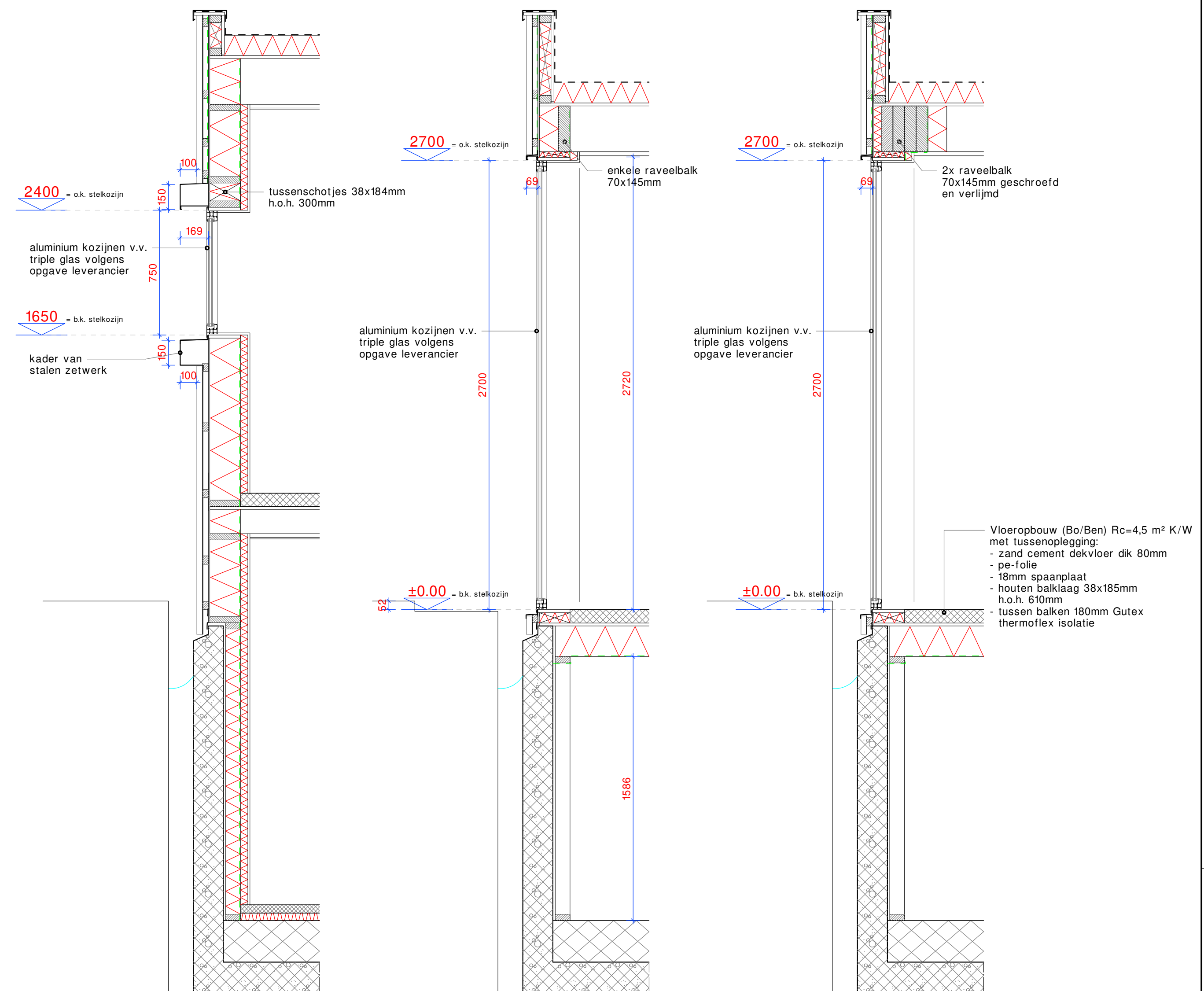
Drasn. B
