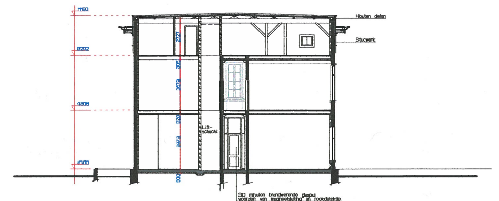
DOORSNEDE A.A.
