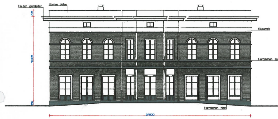
ACHTERGEVEL
