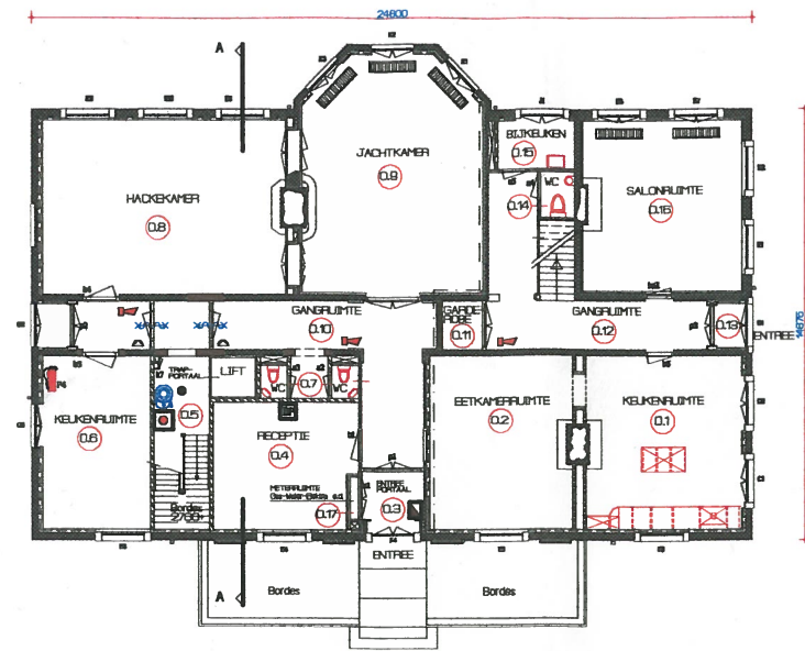
BEGANE GROND
