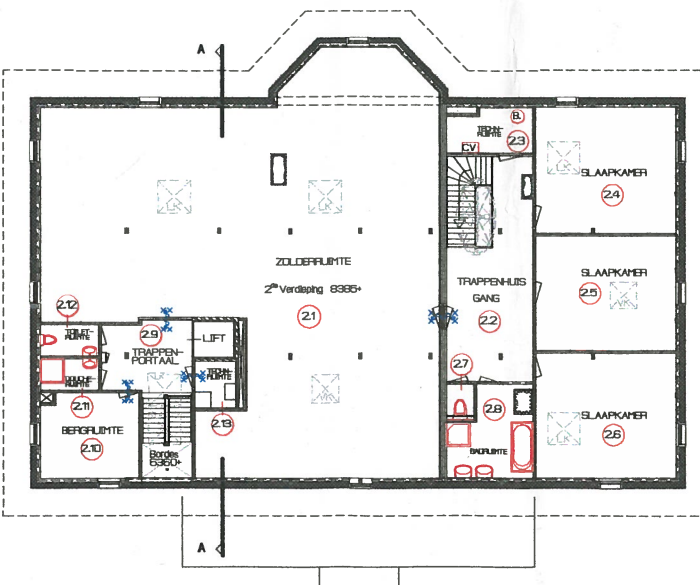
2e VERDIEPING
