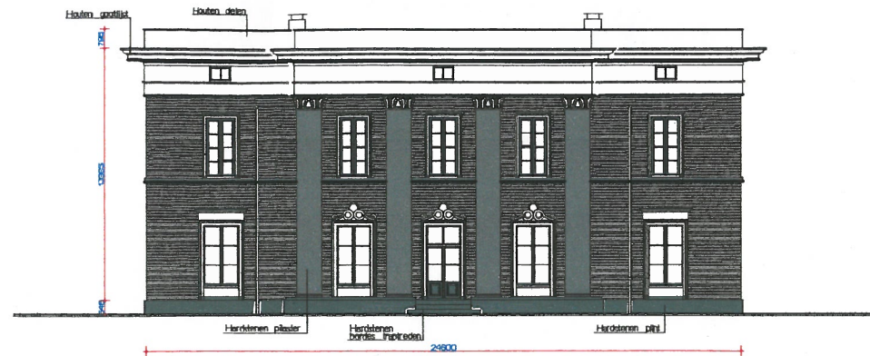
VOORGEVEL
