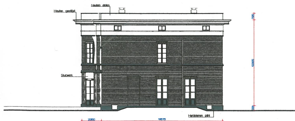
LINKER ZIJGEVEL
