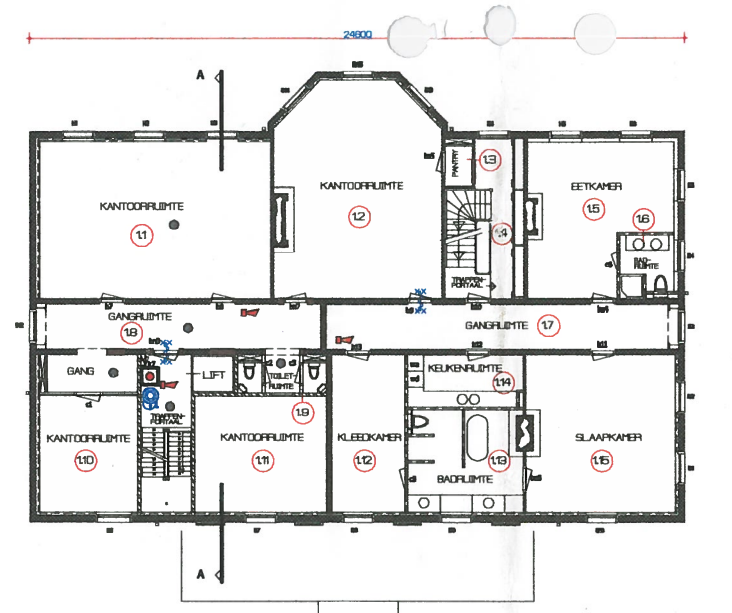
1e VERDIEPING
