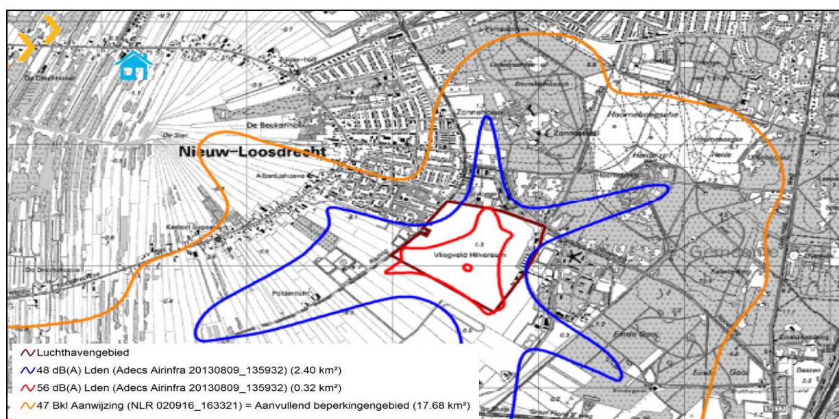
Figuur 2: Geluidscontouren van Vliegveld Hilversum
