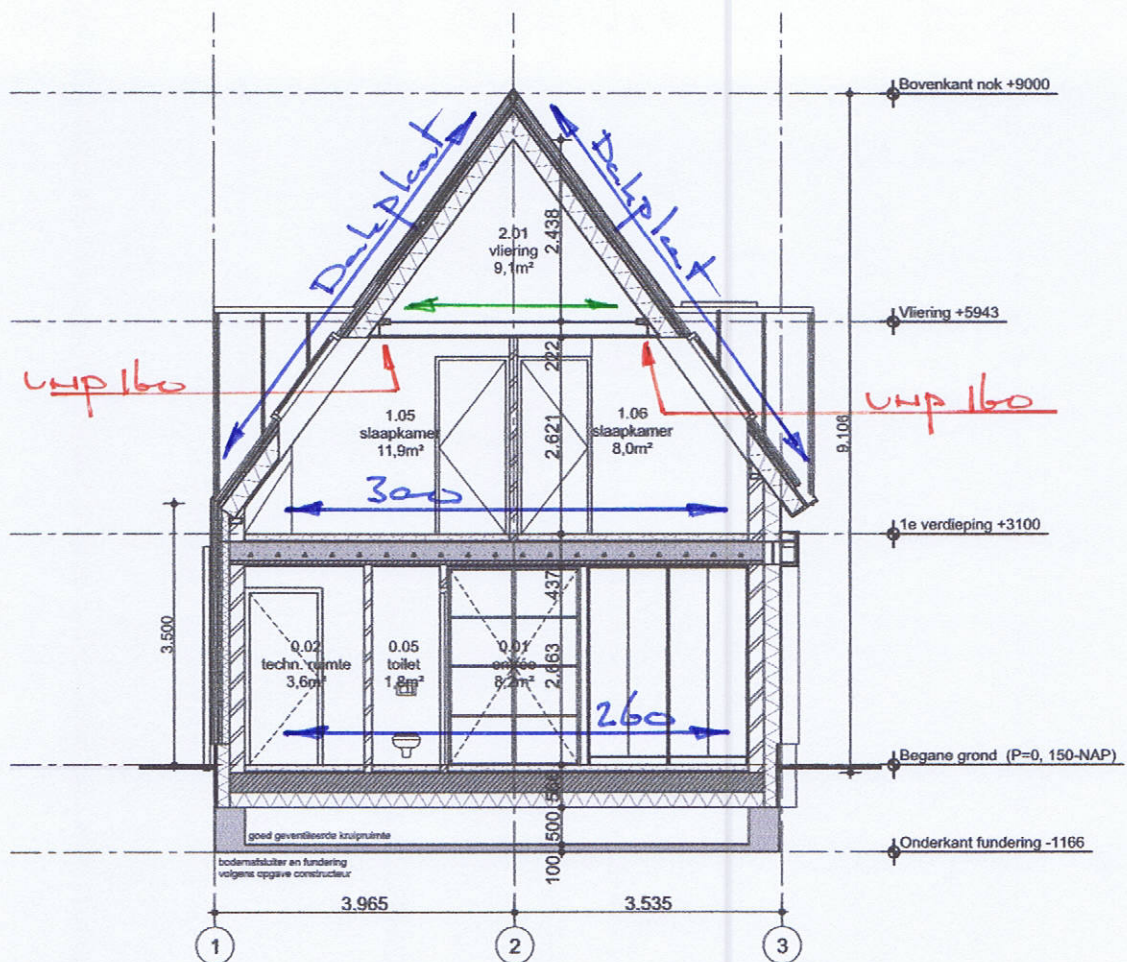
DOORSNEDE A-A
