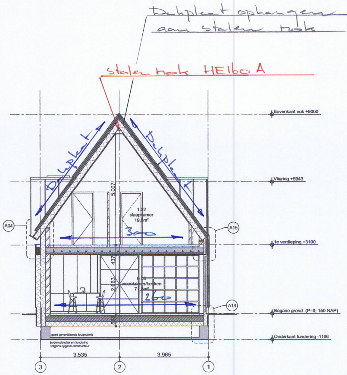
DOORSNEDE F-F
