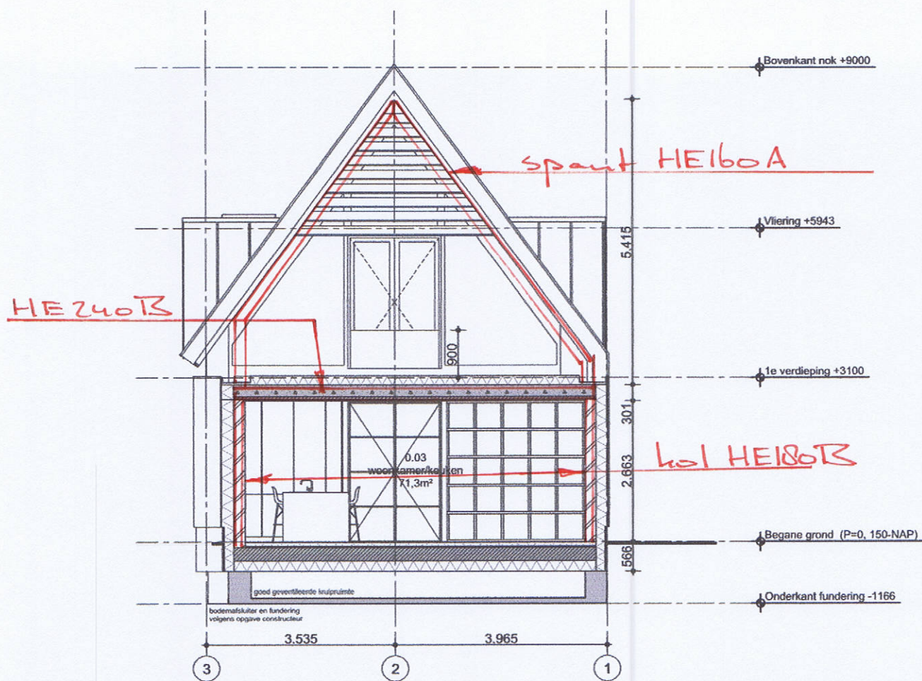
DOORSNEDE C-C
