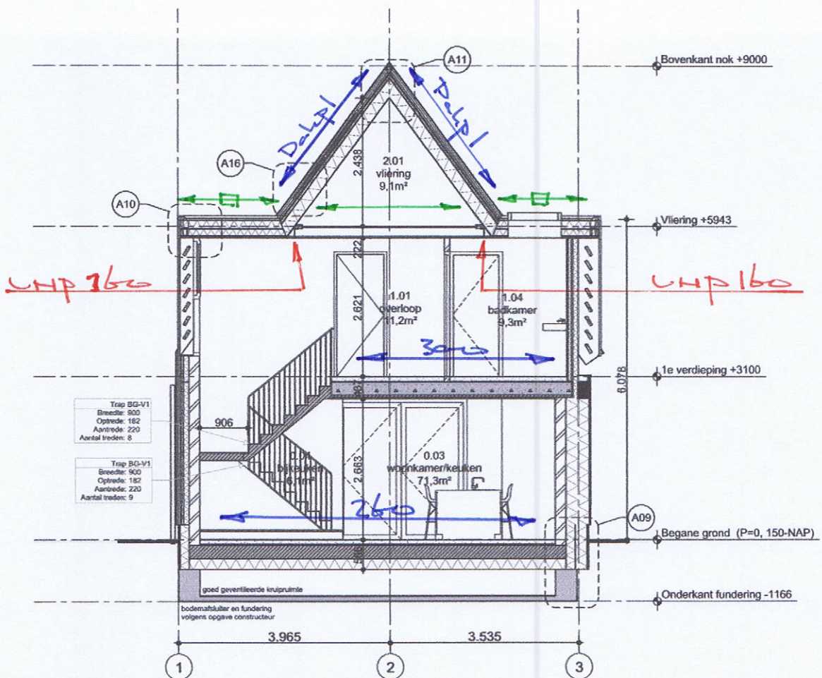
DOORSNEDE B-B
