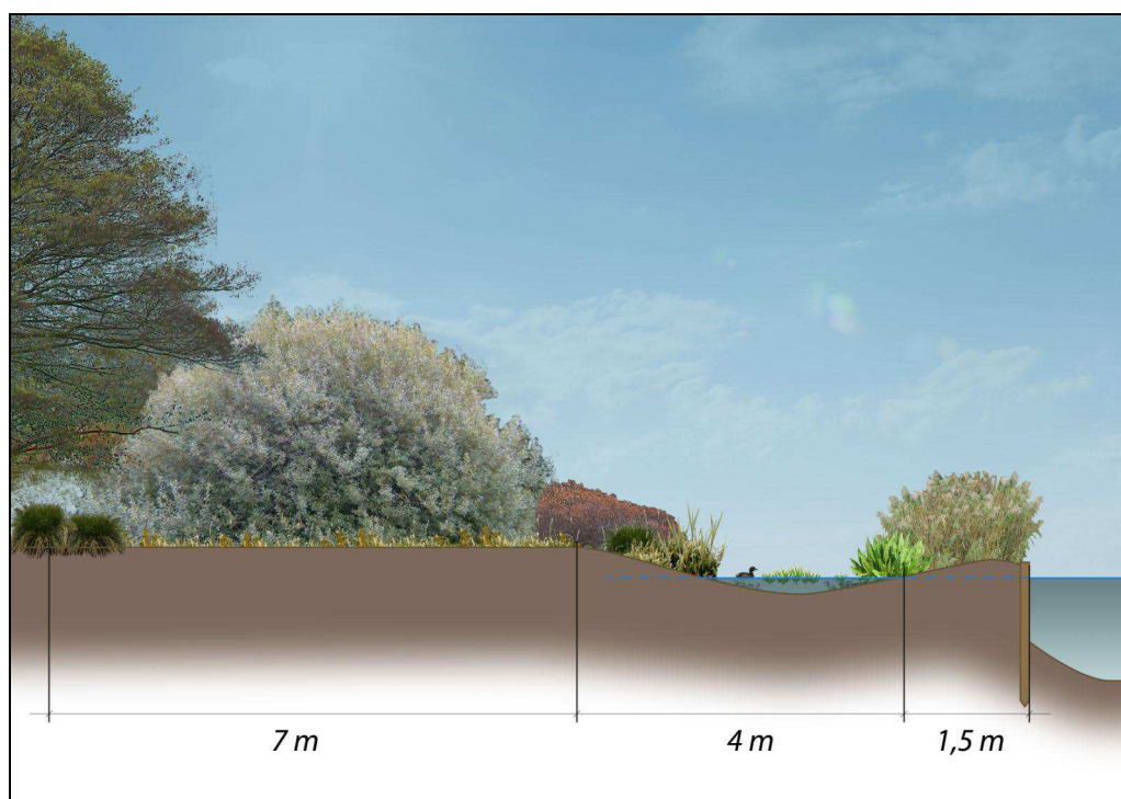
Figuur 5.2 Dwarsdoorsnede natuurvriendelijke oever en struweelrand (A-A')
