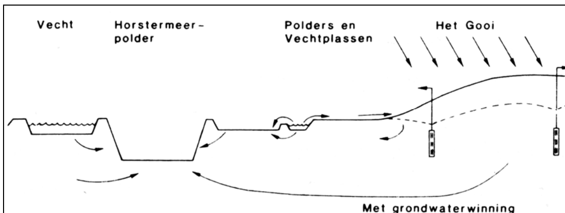
Afbeelding 8 Doorsnede met regionale grondwaterstroming
