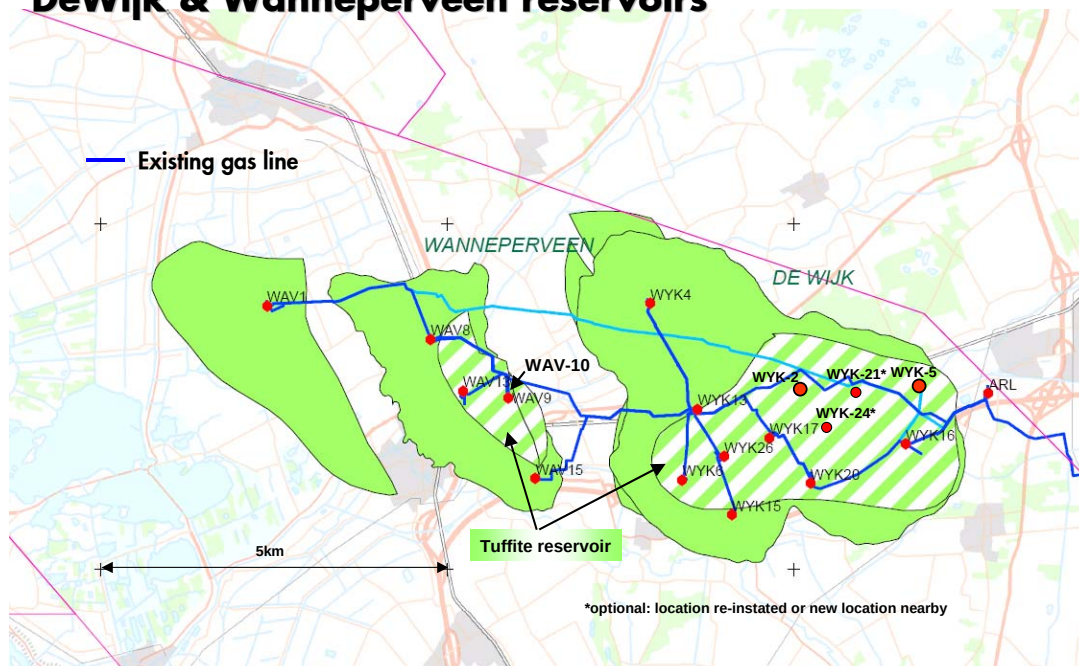
Figuur 3.1 Locatie van put WAV-10, waarin een leak-off test is uitgevoerd voor stikstofinjectie.
