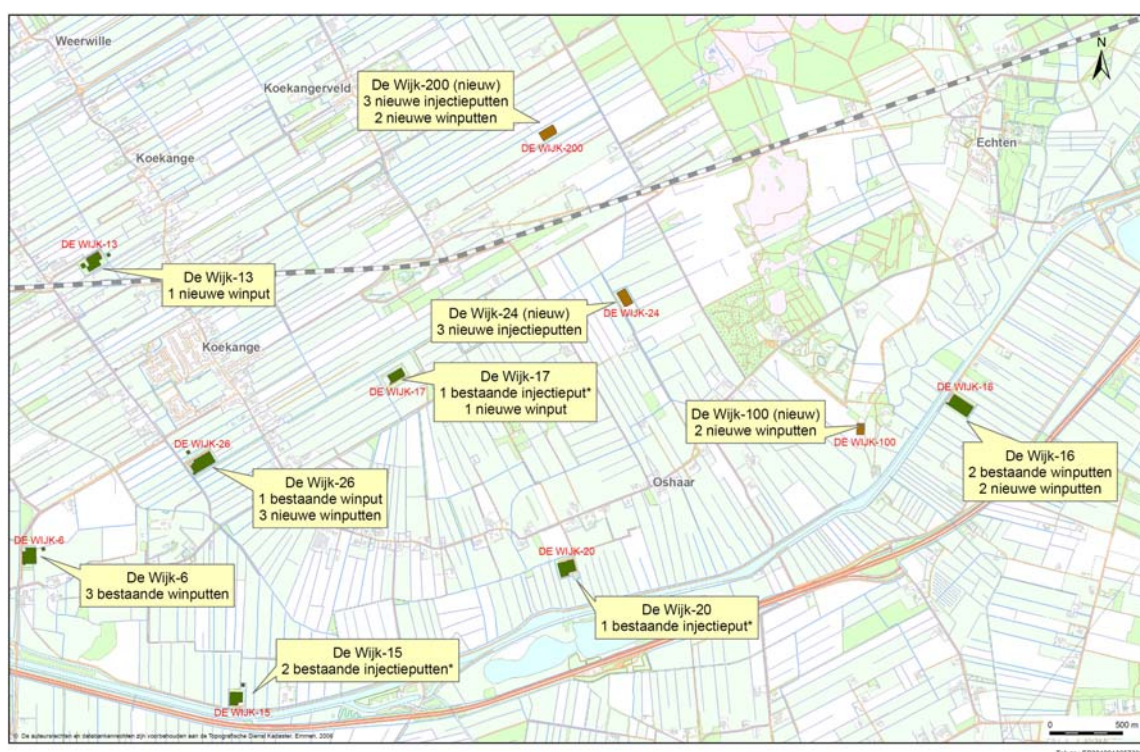
Figuur 4.1 Overzicht locaties en puttenconfiguratie (* winputten worden omgebouwd naar injectieputten)
