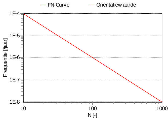
Figuur 12 FN-curve 000669
