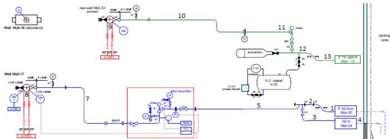
Figuur I- 5: Stromingsdiagram voor De Wijk-17
