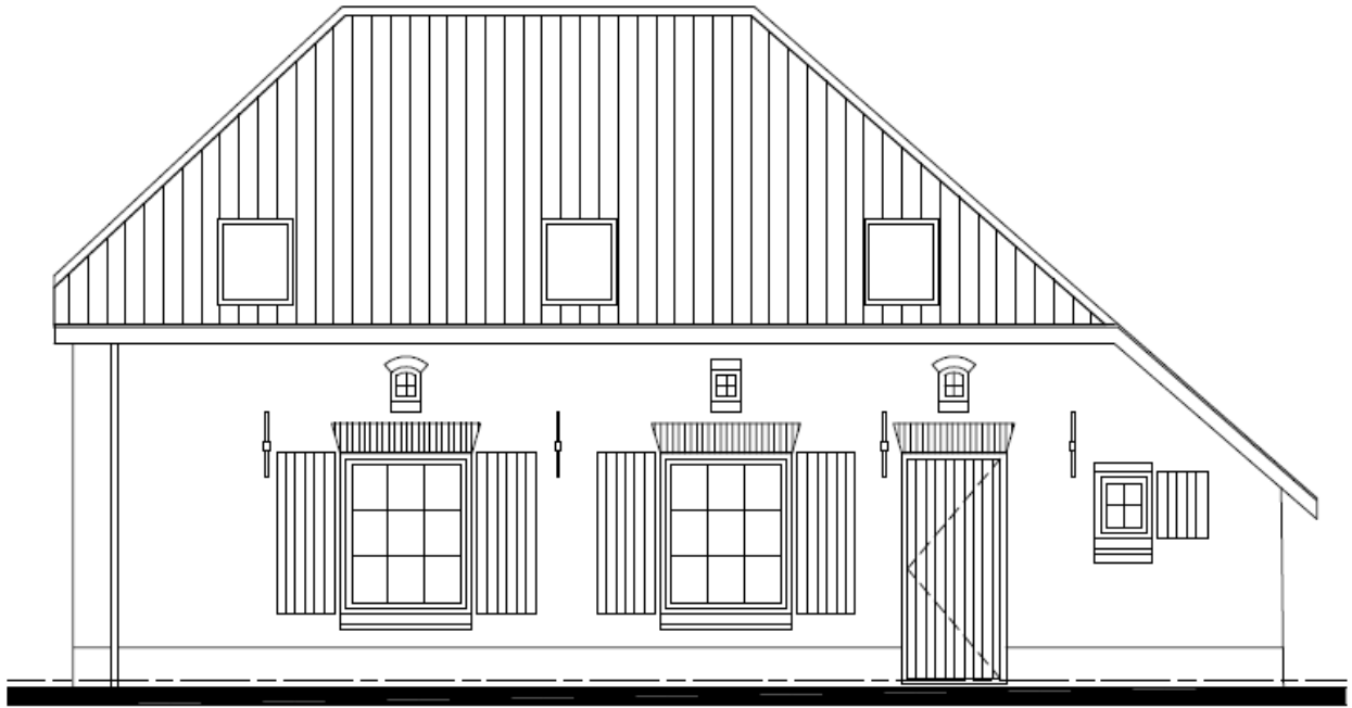
Ontwerp beoogde situatie linker zijgevel
