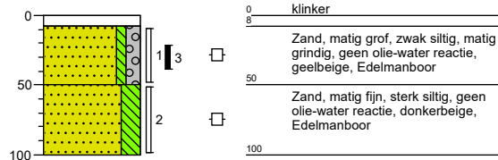
Boring: C03
