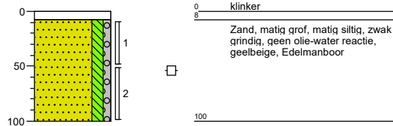
Boring: C01A
