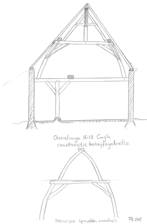
Schets van de bouwhistorisch waardevolle, 18 de -eeuwse houtconstructies van Overhage 16-18. F. Haans 2015
