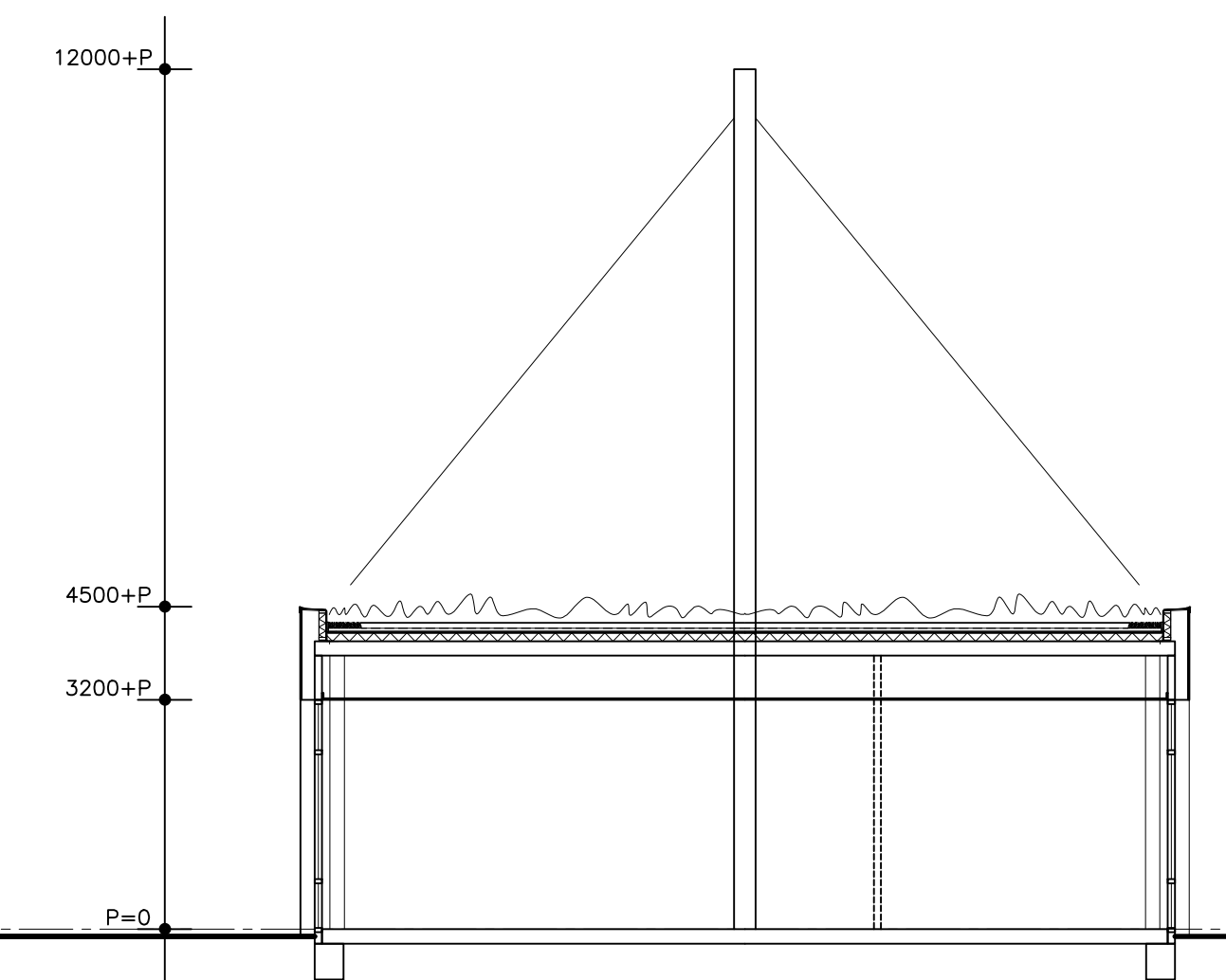
Doorsnede
